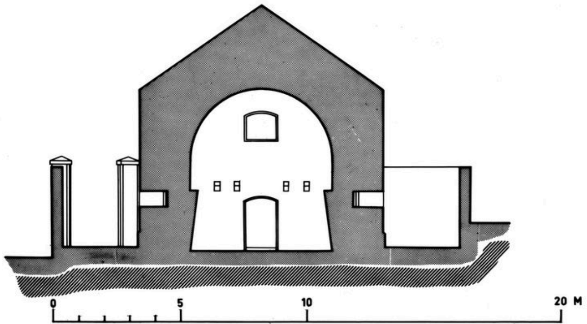
COUPE V.V
