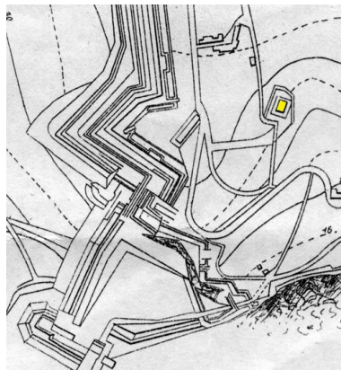
Plan de détail des lignes de Quéléren, Atlas des batteries de côte, 1913. En jaune, l'emplacement du magasin à poudre Repro. Guillaume Lécueillier IVR53_20042903708NUCA
