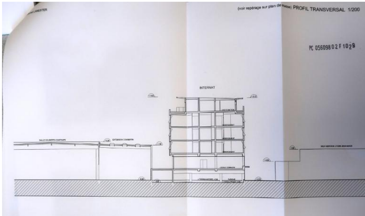
Profil transversal. Agence Déesse 23, architectes, 2002.
