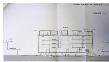
Profil longitudinal. Agence Déesse 23, architectes, 2002. Phot. Thierry Goyet IVR53_20265611093NUCA
