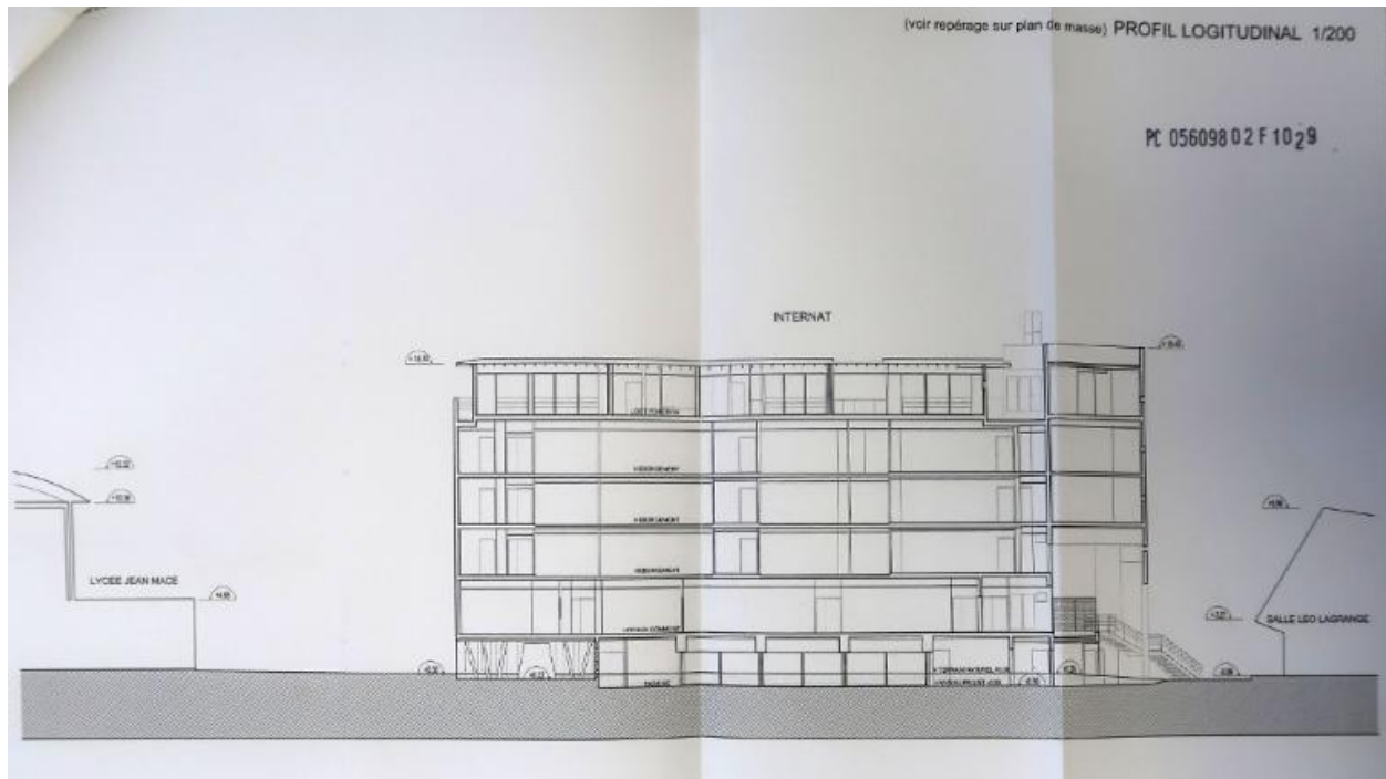
Profil longitudinal. Agence Déesse 23, architectes, 2002.
