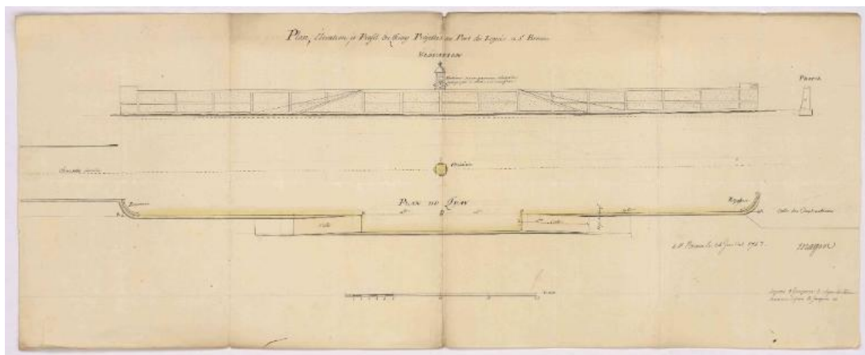
Plan, élévation, profil du quai projeté au port du Légué (1757)
