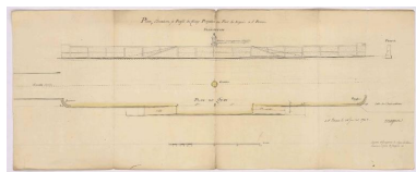
Plan, élévation, profil du quai projeté au port du Légué (1757) Phot. Chocat de Grandmaison, Phot. Magin IVR53_20252210675NUCA
