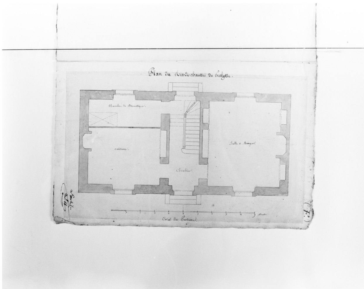
Premier projet signé Lussault, architecte : plan du rez-de-chaussée.
