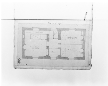
Premier projet signé Lussault, architecte : plan de l'étage. Phot. Bernard Bègne, Autr. architecte Lussault IVR53_19975600269XB
