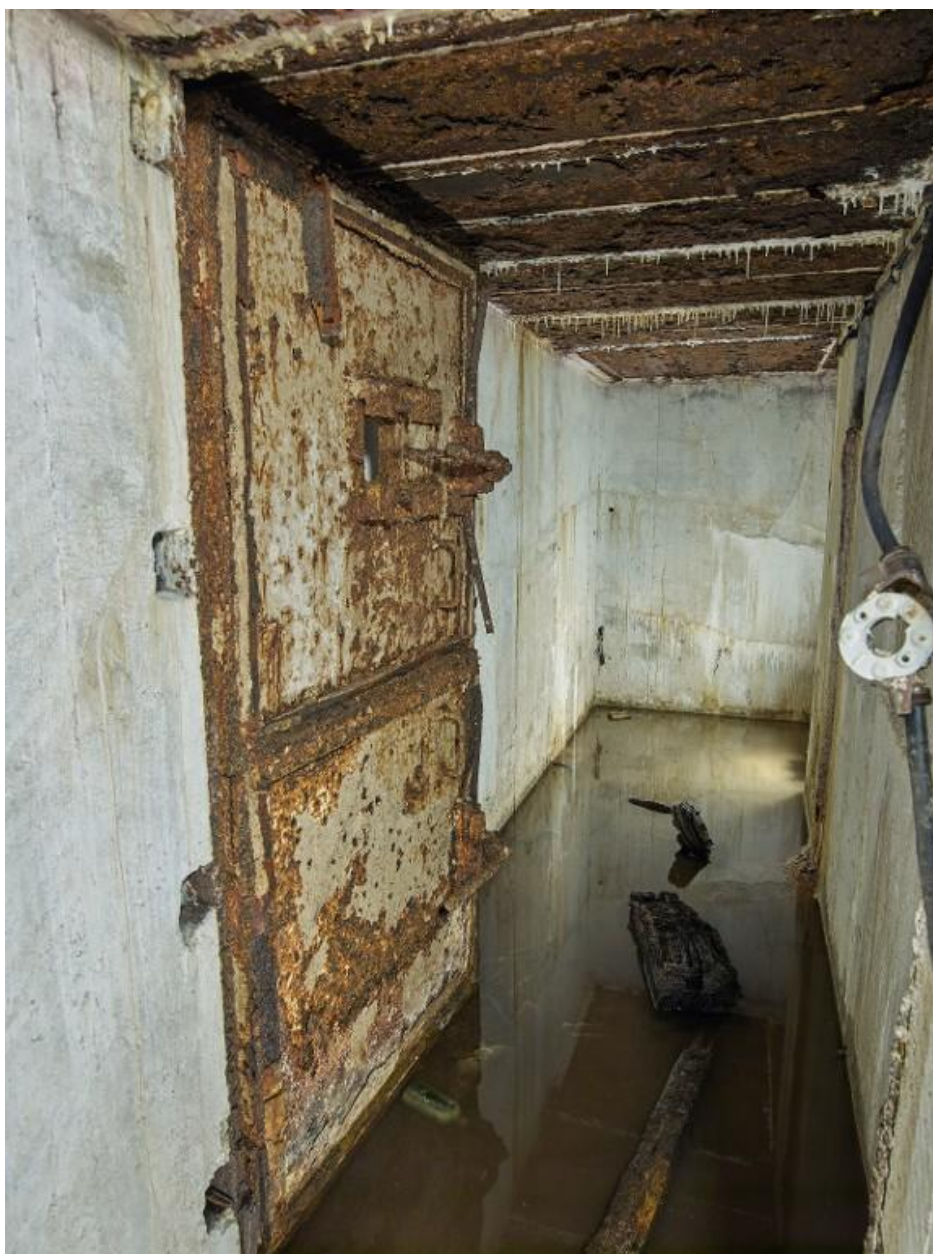
Vue du couloir d'accès de la chambre de combat nord-ouest : porte blindée à deux vantaux. La chambre de combat nord-ouest est partiellement inondée
