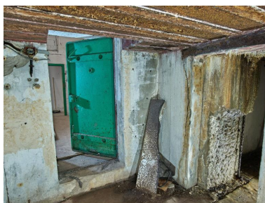
Vue du vestibule avec sa porte étanche. A droite, le mur en béton est élargi afin de permettre un passage plus aisé Phot. Bernard Bègne IVR53_20235600707NUCA
