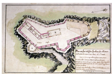
Plan du fort de l'île Herbou (Harbour), fin 17e siècle-début 18e siècle Repro. Guy Artur, Repro. Norbert Lambart
