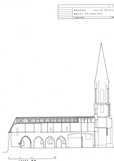
Coupe longitudinale Nord-Sud. Repro. Guy Artur, Repro. Norbert Lambart IVR53_19843500216P
