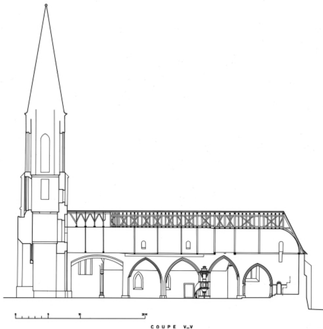
Coupe longitudinale Sud-Nord.
