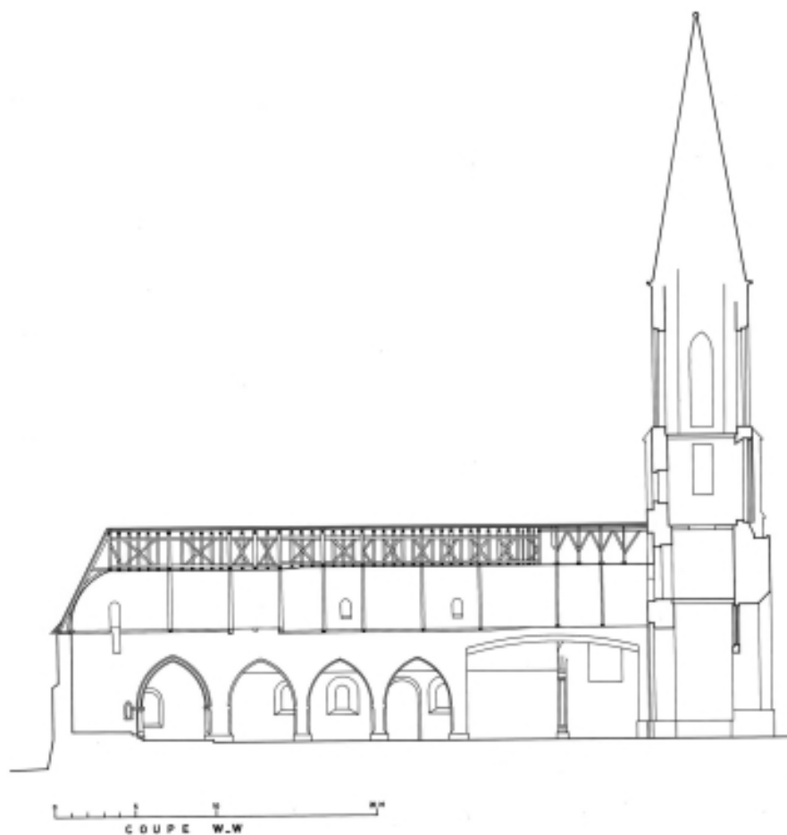
Coupe longitudinale Nord-Sud.
