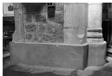
Chœur, base de la 5ème pile. Phot. Guy Artur IVR53_19703500365V
