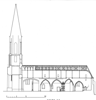
Coupe longitudinale Sud-Nord. Repro. Guy Artur, Repro. Norbert Lambart IVR53_19843500225P
