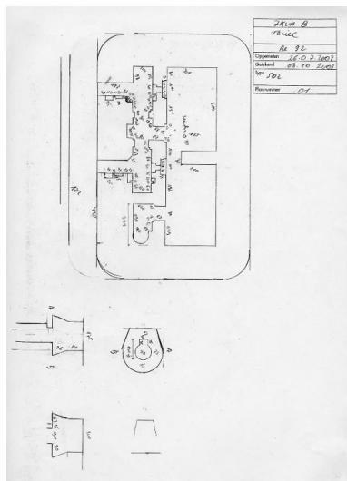
Plan du bunker - abri de type 502 de Tariec (dessin : Dirk Peeters, 2008) Phot. Dirk Peeters IVR53_20242910247NUCA
