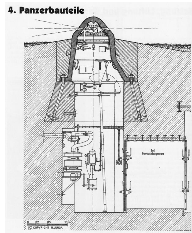
Coupe d'une cloche blindée pour l'observation de l'infanterie (Kleinstglocke für Infanterie-Beobachtung) de type 90P9 (dessin de Robert Jurga extrait de Der Westwall. Geschichte und Gegenwart de Jörg Fuhrmeister, 2004) Phot. Guillaume Lécueillier IVR53_20242910313NUC
