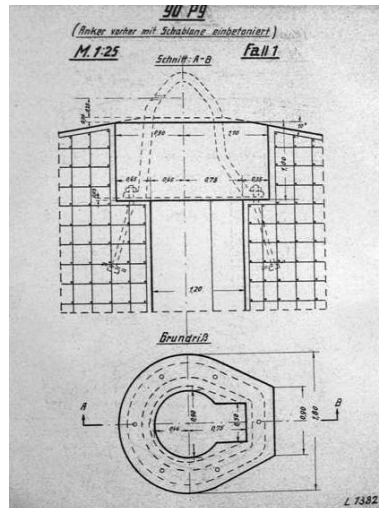
Coupe et plan de la fixation d'une cloche blindée pour l'observation de l'infanterie (Kleinstglocke für Infanterie-Beobachtung) de type 90P9 dans un bunker (extrait du forum Axis history forum, publication de Jopaerya, 2007) Phot. Guillaume Lécueillier IVR53_20242910314NUC
