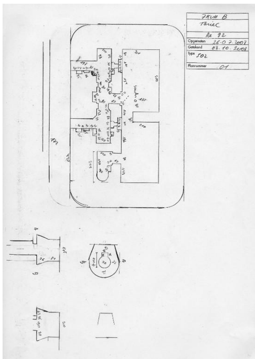
Plan du bunker - abri de type 502 de Tariec (dessin : Dirk Peeters, 2008)
