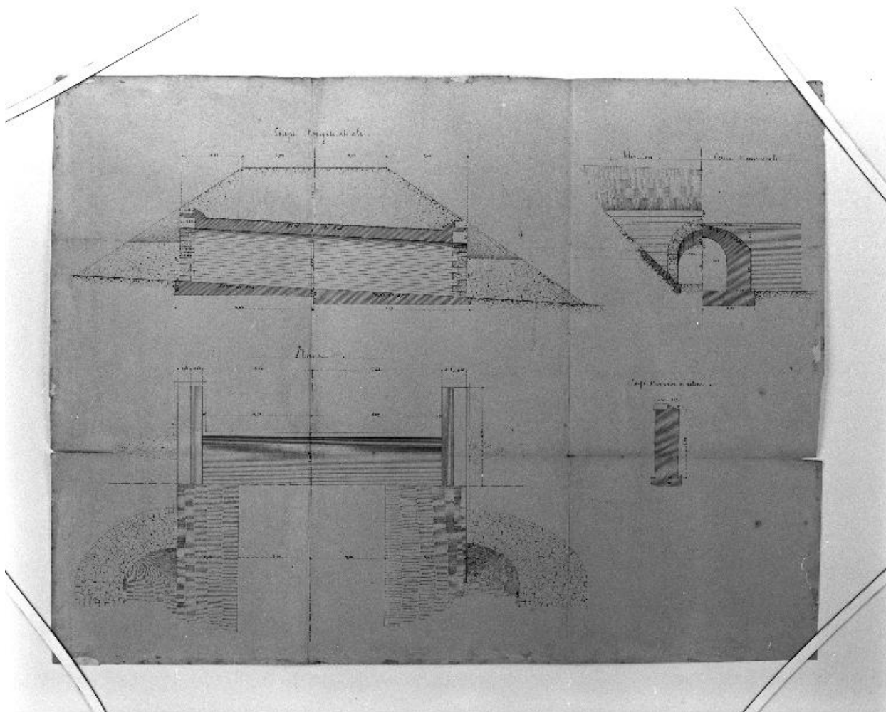
Projet de construction de la partie comprise dans la traversée. Dessin de Ponceau 1869. Coupes longitudinale, transversale, élévation, plan.
