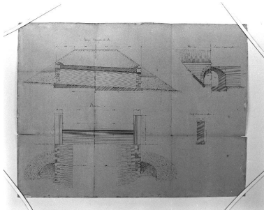
Projet de construction de la partie comprise dans la traversée. Dessin de Ponceau 1869. Coupes longitudinale, transversale, élévation, plan.
