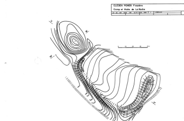
Plan de la motte et de la basse-cour avec courbes de niveau Phot. Auteur inconnu, Phot. A. Beraud IVR53_19672900096V
