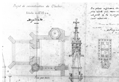
Projet de reconstruction du clocher, plan par terre et plan au niveau AB. Phot. Guy Artur, Phot. Auteur inconnu, Autr. Arthur Regnault IVR53_19953500124V
