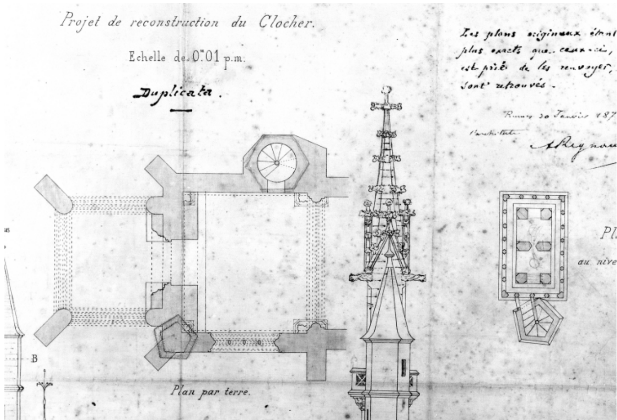
Projet de reconstruction du clocher, plan par terre et plan au niveau AB.
