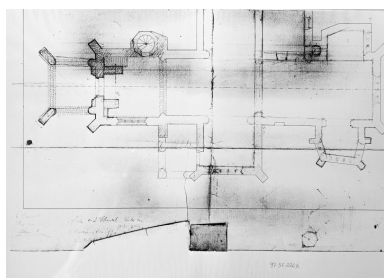
Plan d'implantation du nouveau clocher. A. Regnault Phot. Guy Artur, Phot. Norbert Lambart, Phot. Auteur inconnu, Autr. Arthur Regnault IVR53_19973500226X
