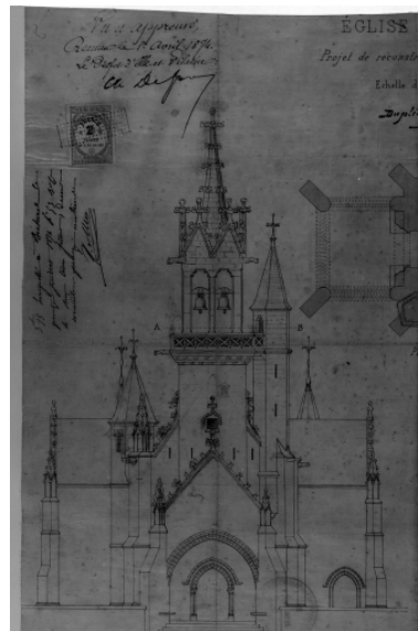
Projet de reconstruction du clocher, vue de face Phot. Guy Artur, Phot. Auteur inconnu, Autr. Arthur Regnault IVR53_19953500123V
