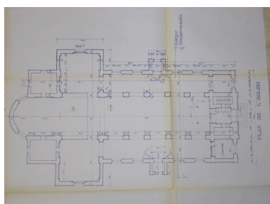
Plonéour-Lanvern, église paroissiale Saint-Eneour : plan au sol Phot. Gwénaél Fauchille IVR53_20082905866NUCA
