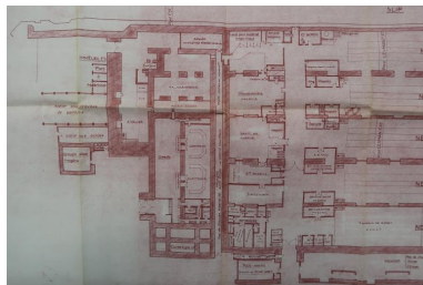
Extrait du plan du bloc n° 1, distribution des locaux : rez-de-chaussée de la centrale électrique, plan K n° 780A, 28 décembre 1965, mis à jour du 11 avril 1979 (Service Historique de la Défense de Lorient) Phot. Guillaume Lécueillier IVR53_20235605340NUCA
