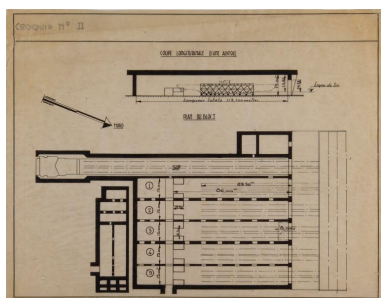
Plan et coupe longitudinale du bunker "KI", croquis II (Service Historique de la Défense de Lorient, Monographie de la base "Ingénieur Général Stosskopf", 1945-1946) Phot. Service Historique de la Défense IVR53_20225606354NUCA
