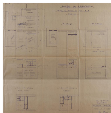
Plan du bunker pour machines, plan K n° 8 bis, 17 janvier 1945 (Service Historique de la Défense de Lorient, Monographie de la base "Ingénieur Général Stosskopf", 1945-1946) Phot. Service Historique de la Défense
