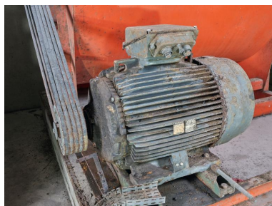
Vue de la salle des ventilateurs : moteur électrique de la Compagnie Electro-Mécanique entraînant via des courroies un ventilateur industriel de marque Fevi. Les fils d'alimentation ont été coupés Phot. Bernard Bègne IVR53_20235600231NUCA
