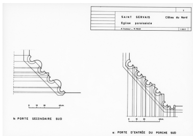
Profil des moulures, porte secondaire sud, porte d'entrée porche sud Phot. François Dagorn IVR53_19762200091P
