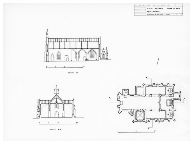
Plan et coupes Phot. François Dagorn IVR53_19762200090P
