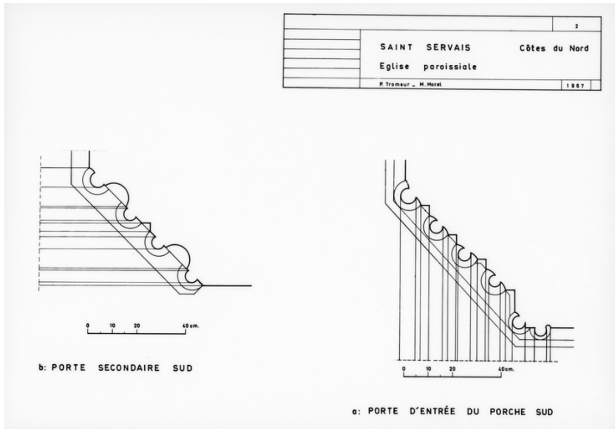
Profil des moulures, porte secondaire sud, porte d'entrée porche sud
