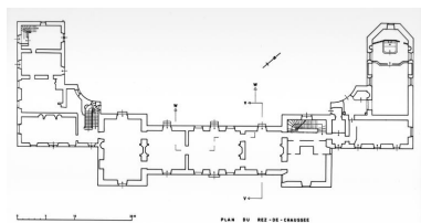
Plan du rez-de-chaussée. Phot. Service régional de l'Inventaire de Bretagne IVR53_19863500922P
