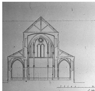
Coupe transversale du chevet. Phot. Guy Artur, Phot. Norbert Lambart, Autr. Arthur Regnault, Autr. Aristide Tourneux IVR53_19973500045X
