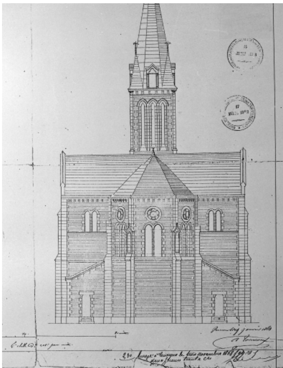
Elévation du chevet de l'église
