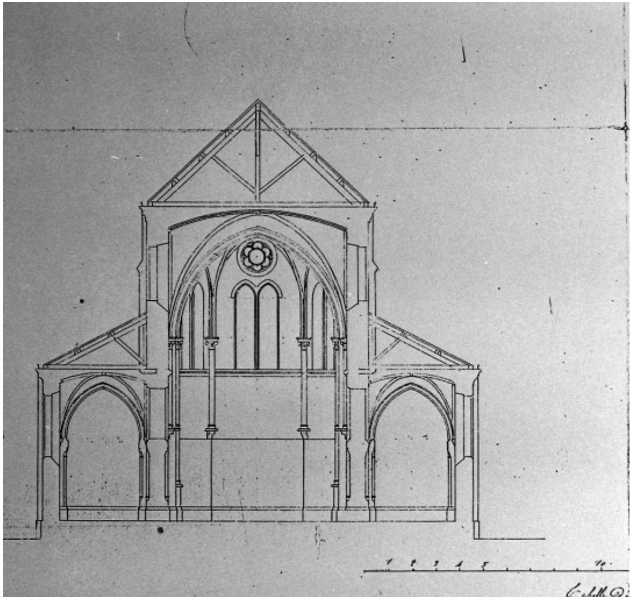
Coupe transversale du chevet.
