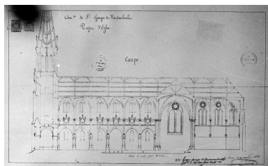
Projet d'église, coupe. Phot. Guy Artur, Phot. Norbert Lambart, Autr. Arthur Regnault, Autr. Aristide Tourneux IVR53_19973500047X
