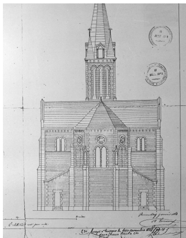
Elévation du chevet de l'église Phot. Guy Artur, Phot. Norbert Lambart, Autr. Arthur Regnault, Autr. Aristide Tourneux IVR53_19973500046X
