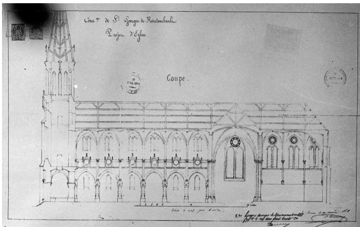
Projet d'église, coupe.
