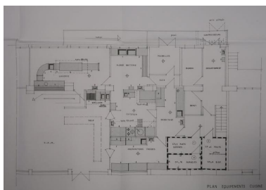
Restructuration des cuisines : plan. Pascal Debard, architecte, 1998-1999. Autr. Pascal Debard IVR53_20215605018A0
