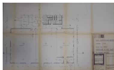
Construction de trois salles de travaux pratiques : plan. Michel Ysvelain et Claude Blin, architecte, 1985. Autr. Michel Ysvelain, Dess. Claude Blin IVR53_20215605026A2
