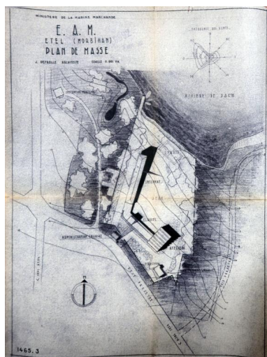
Plans de masse l'E.A.M. (école d'apprentissage maritime) - Etel. Jacques Deyrolle, architecte, sd. Plan de masse correspondant aux plans des bâtiments datés du 23 mai 1952. Autr. Jacques Deyrolle
