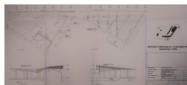
Restructuration du bâtiment A3 : plan du nouveau préau et de la classe de navigation. Pascal Debard, architecte, 1998-1999. Autr. Pascal Debard IVR53_20215605014A0
