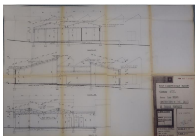
Construction de trois salles de travaux pratiques : coupes. Michel Ysvelain et Claude Blin, architecte, 1985. Autr. Michel Ysvelain, Dess. Claude Blin IVR53_20215605024A0
