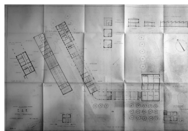
Plans de l'E.A.M. (école d'apprentissage maritime) - Etel. Jacques Deyrolle, architecte, 23 mai 1952. Autr. Jacques Deyrolle IVR53_20215605006A0
