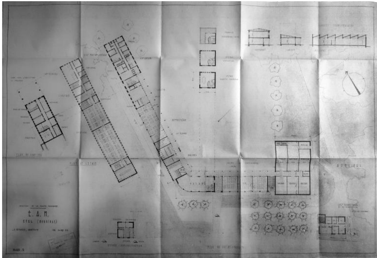
Plans de l'E.A.M. (école d'apprentissage maritime) - Etel. Jacques Deyrolle, architecte, 23 mai 1952.
