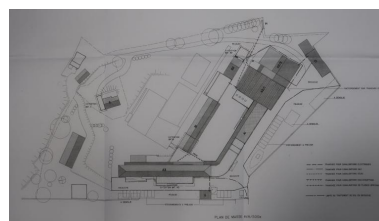
Restructuration de 1998 : plan de masse. Pascal Debard, architecte, 1998-1999. Autr. Pascal Debard IVR53_20215605015A0
