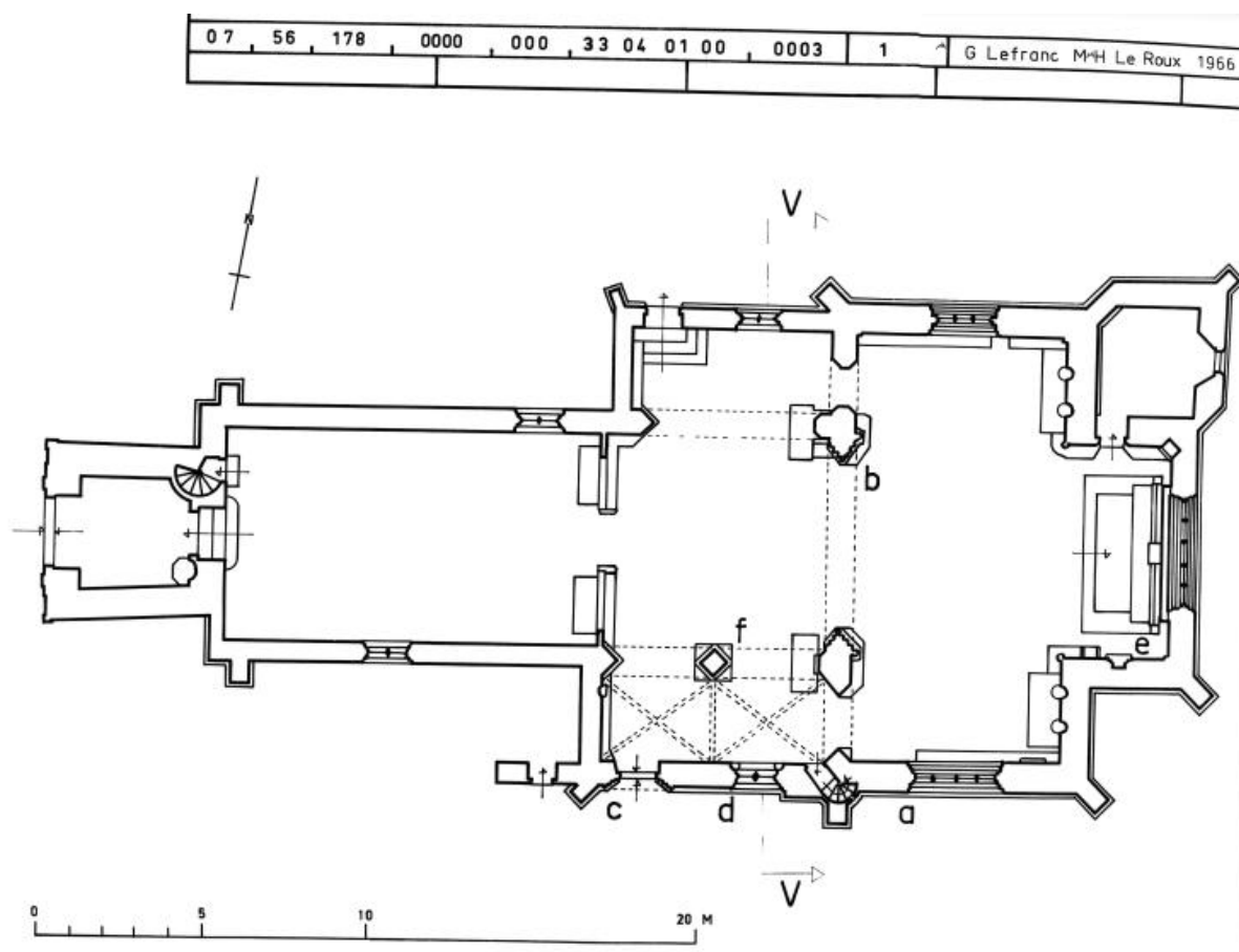
Plan au sol
