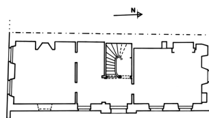
PLAN DU REZ-DE-CHAUSSEE
