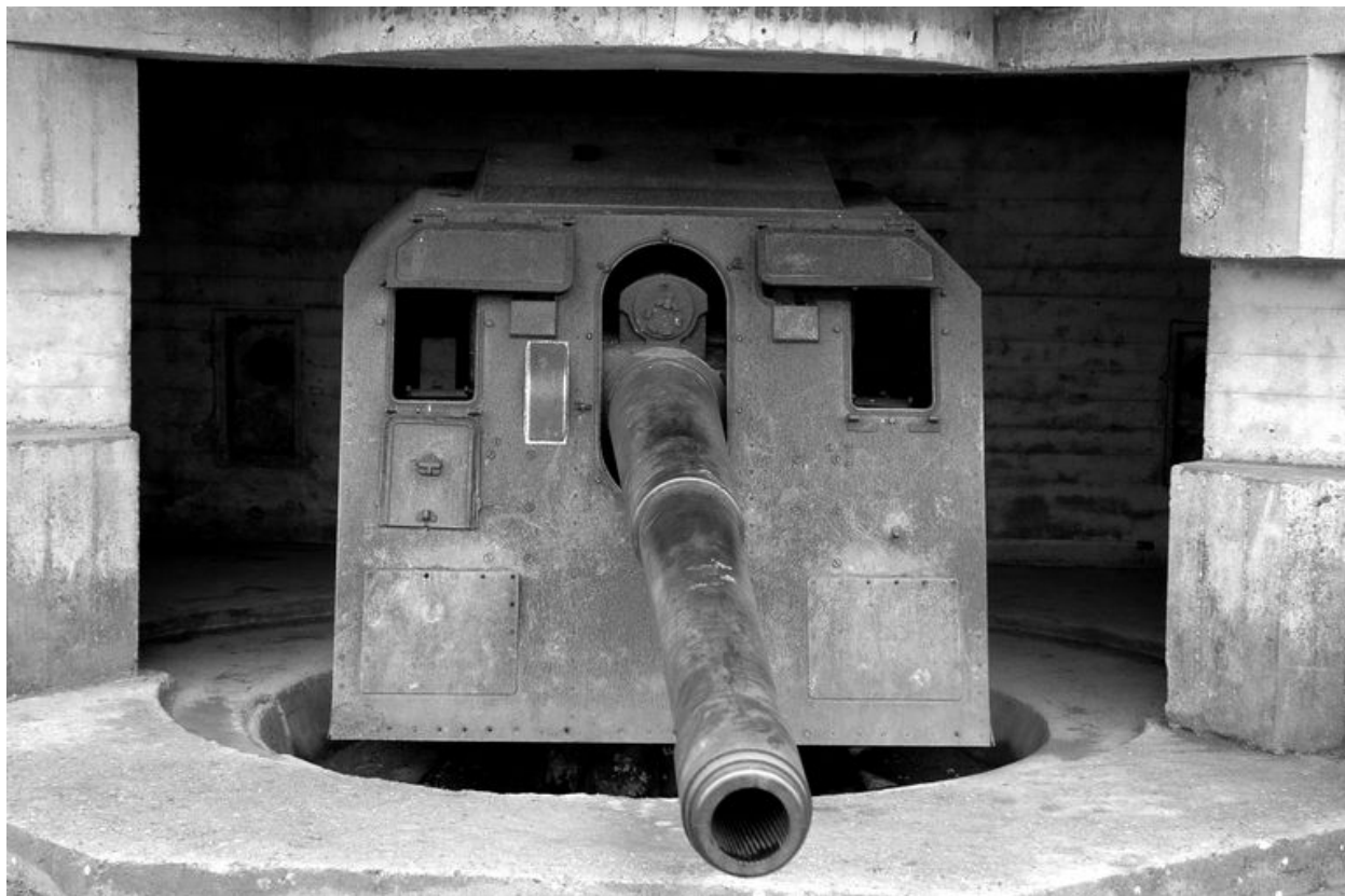
Vue de la tourelle de canon de l'une des quatre casemates de la batterie de Longues-sur-Mer (casemate n° 4 depuis l'est)
