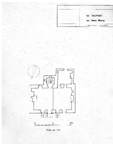
Maison : plan au sol du rez-de-chaussée (état en 1985) Autr. Philippe Boutroux, Autr. Corinne Lerebour IVR53_19855600892P
