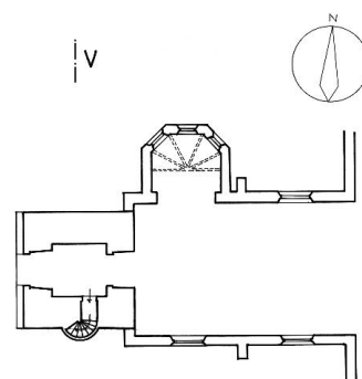
PLAN REZ DE CHAUSSEE 0 5 10m
