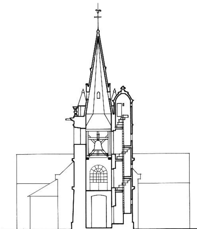
COUPE V V' VERS L'EST
