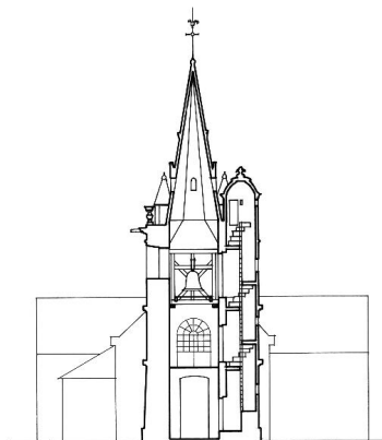
COUPE VV' VERS L'EST 0 5 10m
