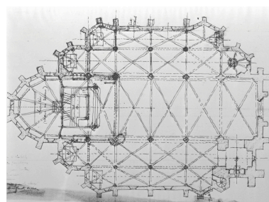
Avant projet de l'église par Arthur Regnault Repro. Guy Artur, Repro. Norbert Lambart IVR53_19973500294X
