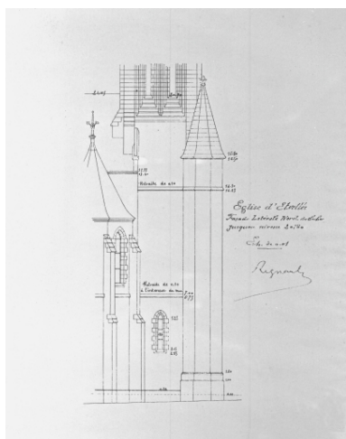
Élévation, détail Repro. Guy Artur, Repro. Norbert Lambart IVR53_19973500297X
