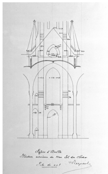
Elévation du clocher, détail Repro. Guy Artur, Repro. Norbert Lambart IVR53_19973500296X
