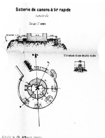
Plans et coupes des batterie casematée et à tir rapide, 1893 : détail de la batterie à tir rapide (Direction d'Artillerie du génie de Brest, colonel directeur d'Artillerie Collomb) Phot. Guy Artur, Phot. Norbert Lambart, Autr. IVR53_20052904172NUCA
