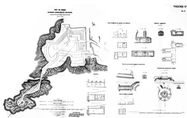
Plans et coupes des batterie casematée et à tir rapide, 1893 (Direction d'Artillerie du génie de Brest, colonel directeur d'Artillerie Collomb) Phot. Guy Artur, Phot. Norbert Lambart, Autr. IVR53_19702900074Z
