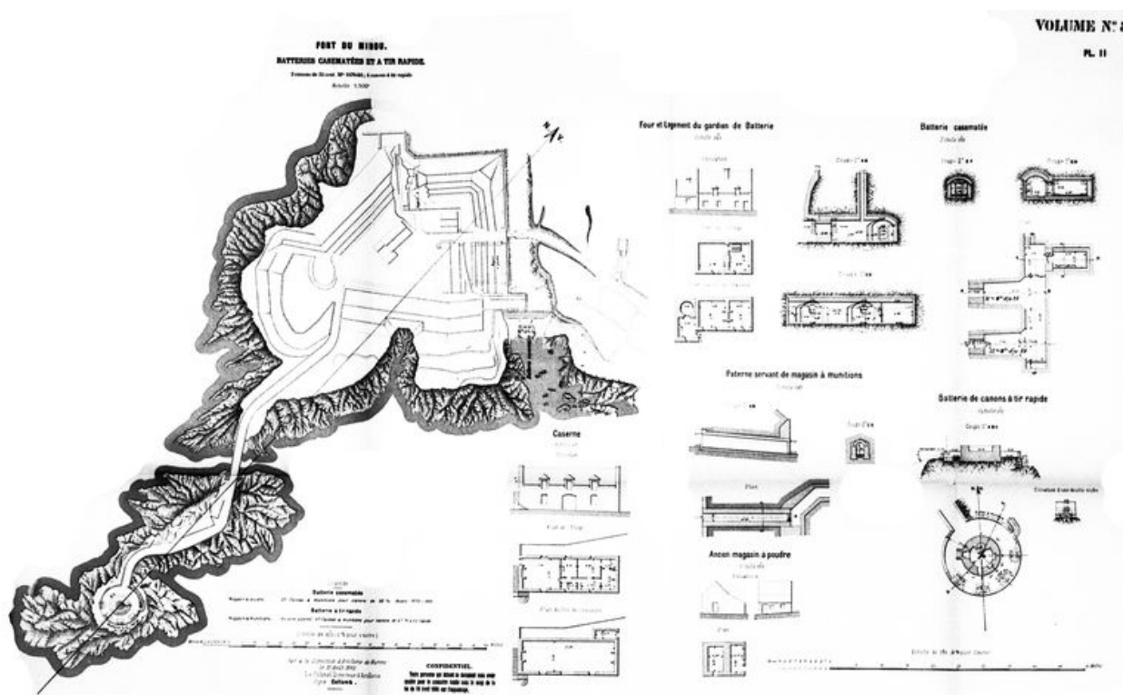
Plans et coupes des batterie casematée et à tir rapide, 1893 (Direction d'Artillerie du génie de Brest, colonel directeur d'Artillerie Collomb)
