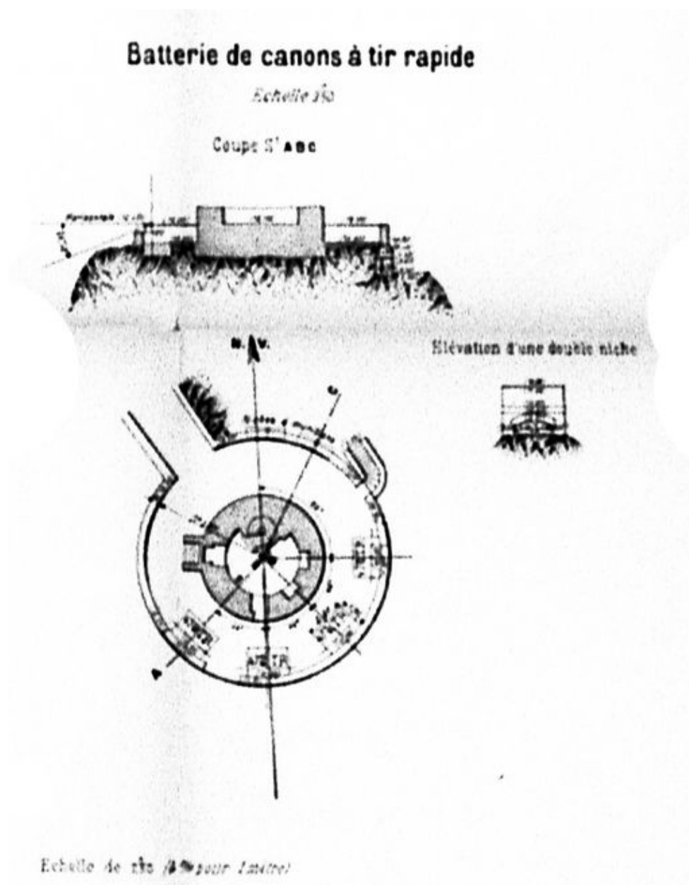
Plans et coupes des batterie casematée et à tir rapide, 1893 : détail de la batterie à tir rapide (Direction d'Artillerie du génie de Brest, colonel directeur d'Artillerie Collomb)
