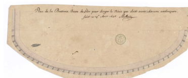
Plan de la batterie de Léon, fait à Brest le 24 août 1686 par Mollart. Plan de la batterie basse de Léon pour diriger le biais que doit avoir chacune embrasure Repro. Service Historique de la Défense, Autr. Paul-Louis Mollart IVR53_20082908836NUCA
