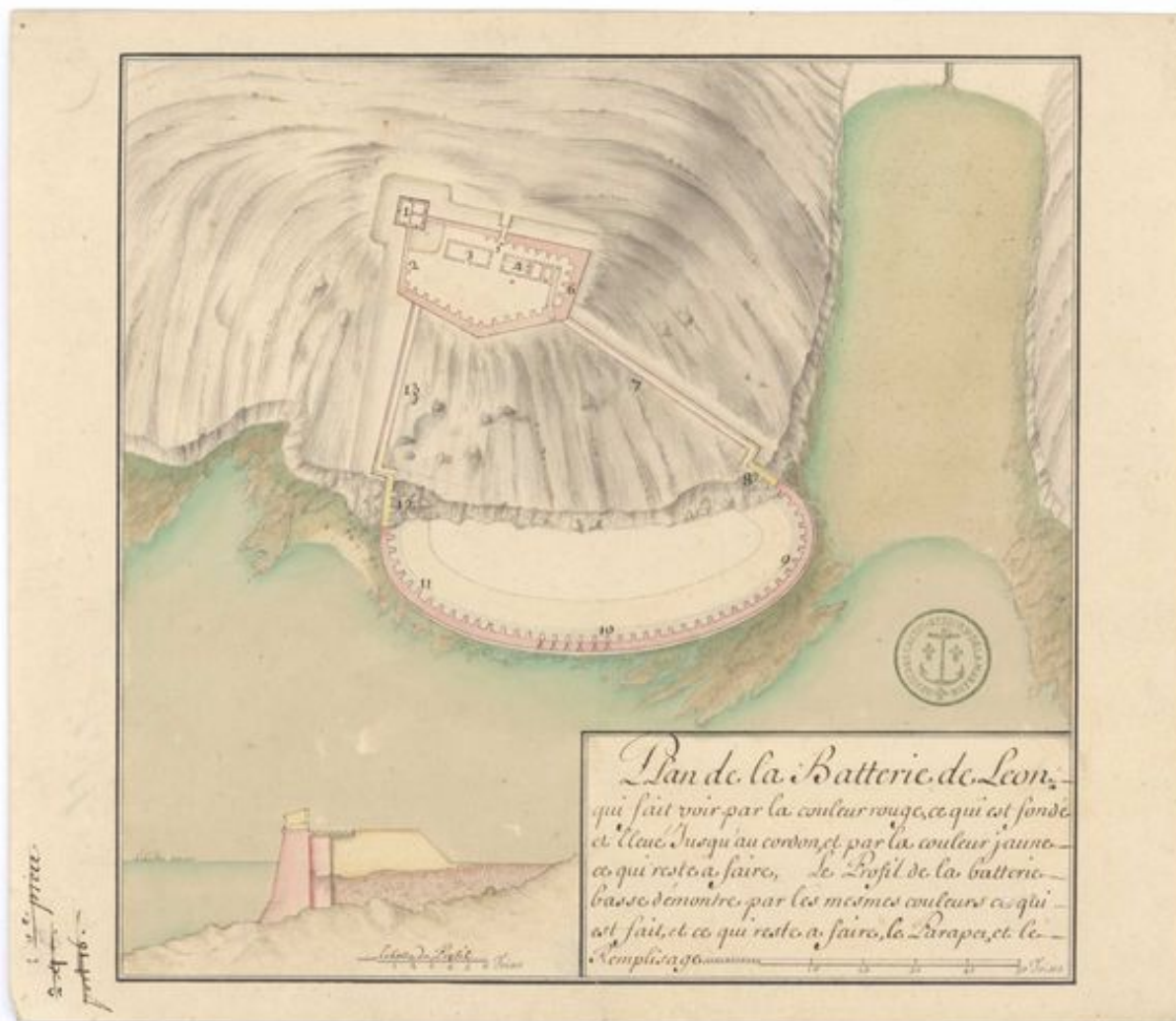
Plan de la batterie de Léon, fait en 1686 par Mollart. Plan général et profil des projets pour 1687
