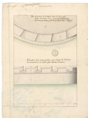
Plan de la batterie de Léon, fait à Brest le 24 août 1686 par Mollart. Plan et élévation d'une partie de la batterie basse : pour diriger l'ouverture de ses embrasures ; pour diriger la hauteur du revêtement au dessus des plus hautes marées
