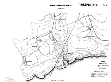
Plan d'ensemble du fort du Mengant et batteries extérieures, Direction d'Artillerie du génie de Brest, 10 août 1893, par le colonel Directeur d'Artillerie : Collomb Repro. Guy Artur, Repro. Norbert Lambart, Autr. IVR53_19702900075Z
