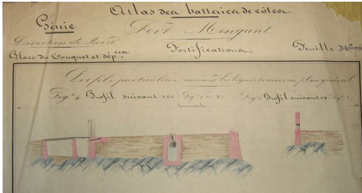
Plan du fort du Mengant : détail du pont-levis, profil suivant A-B-C et C-D, Atlas des batteries de côte, Génie, Direction de Brest, 1839 par Narjot
