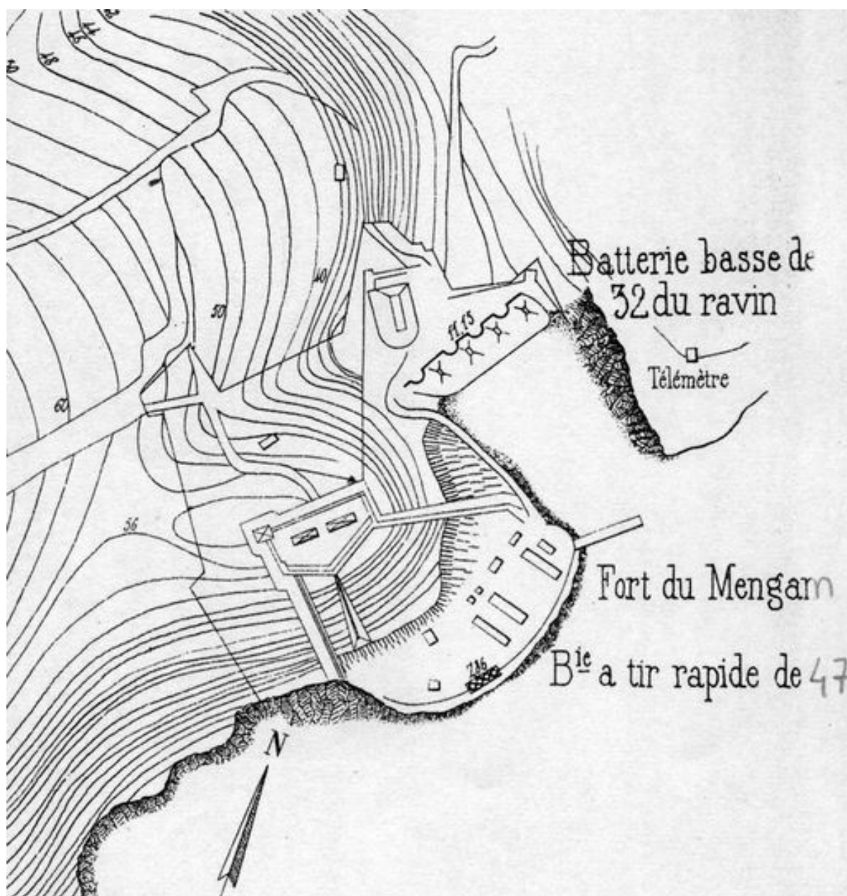
Détail du plan de situation des batteries du Mengant (batterie du fort : canons à tir rapide de 47 mm, batterie basse du ravin : 4 canons de 32 cm), Atlas des batteries de côte : côte de Brest, 1913, Vincennes
