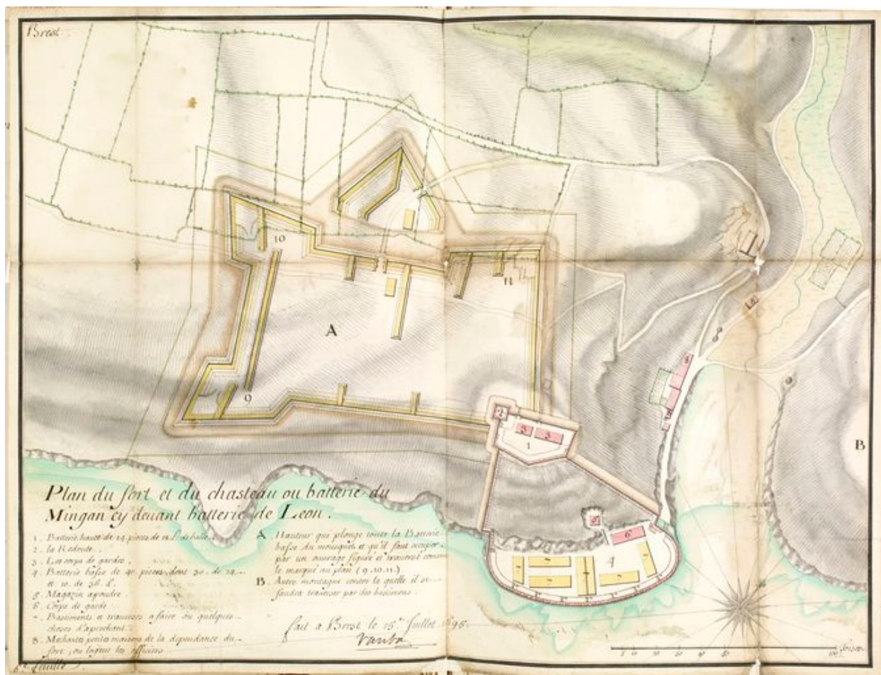
Plan du fort du Mengant et de la batterie de Léon, fait à Brest le 15 juillet 1695 et signé par Vauban. Bibliothèque du Génie, Manuscrit in f°33g tome 2 atlas
