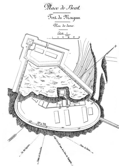
Plan du fort du Mengant (batterie du fort : canons à tir rapide de 47 mm), Atlas des batteries de côte : côte de Brest, 1913, Vincennes Repro. Guy Artur, Repro. Norbert Lambart, Autr. IVR53_19702900053Z
