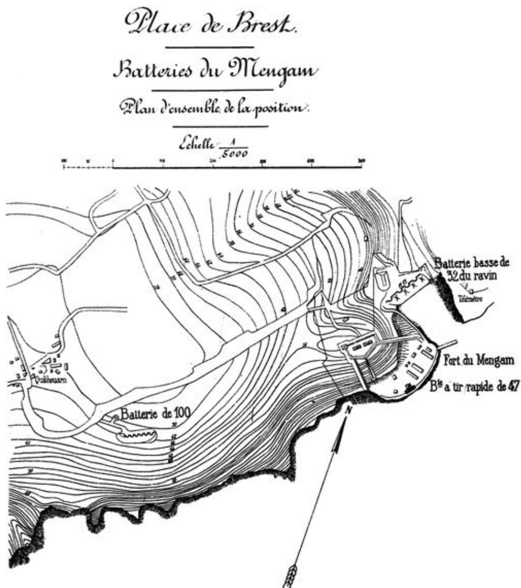
Plan de situation des batteries du Mengant, Atlas des batteries de côte : côte de Brest, 1913
