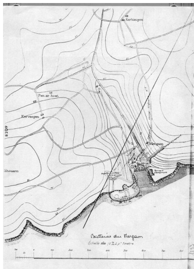
Plan de situation des batteries du Mengant (batterie du fort : canons à tir rapide de 47 mm, batterie basse du ravin : 4 canons de 32 cm), Atlas des batteries de côte : côte de Brest, 1893, Vincennes Repro. Guillaume Lécullier IVR53_20042903699NUCA
