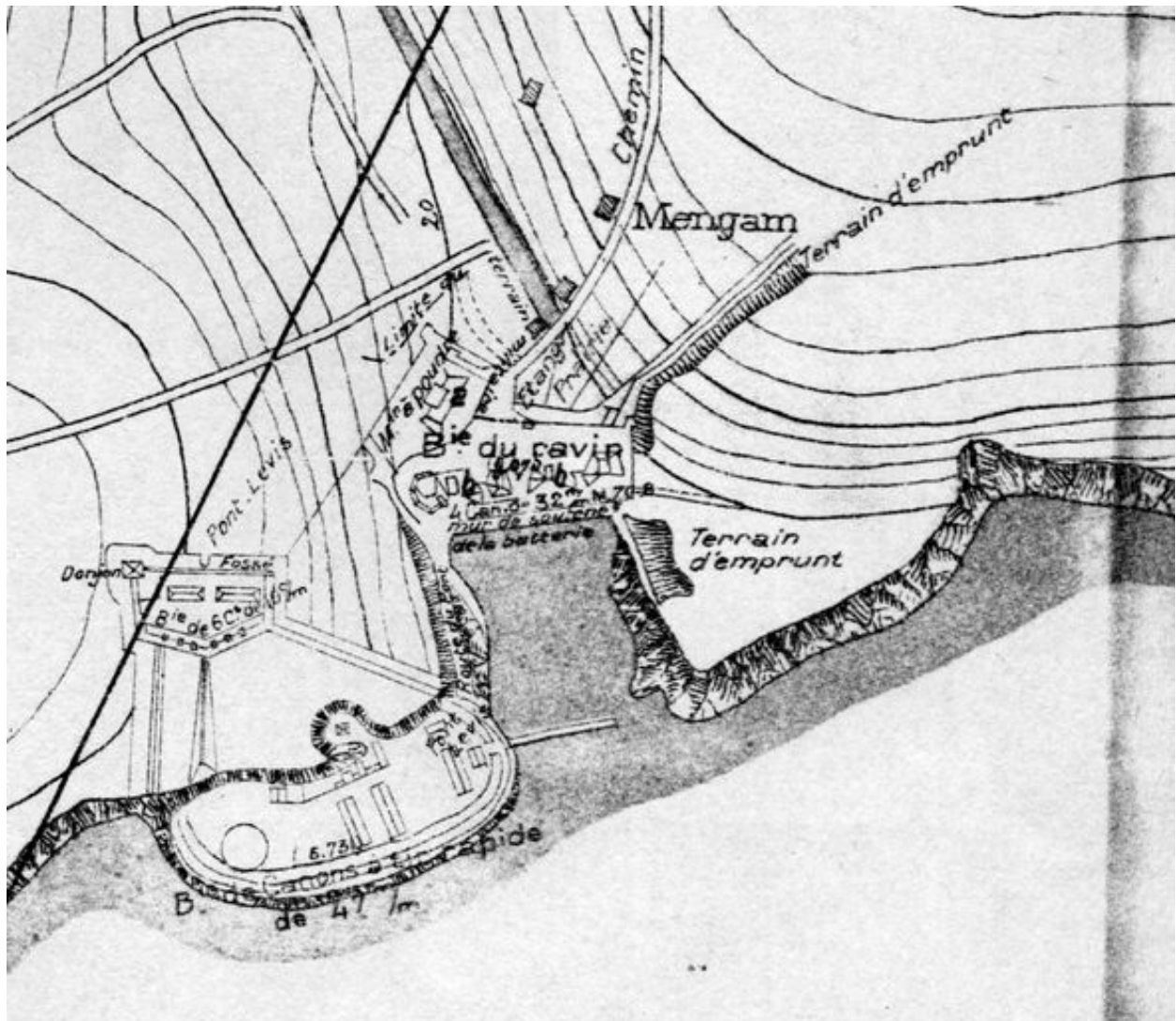
Détail du plan de situation des batteries du Mengant (batterie du fort : canons à tir rapide de 47 mm, batterie basse du ravin : 4 canons de 32 cm), Atlas des batteries de côte : côte de Brest, 1893, Vincennes
