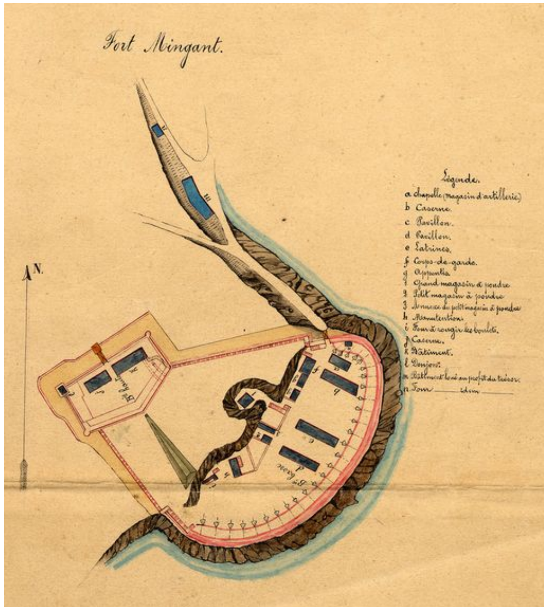
Plan du fort du Mengant, Génie, Direction de Brest, 2e moitié 19e siècle
