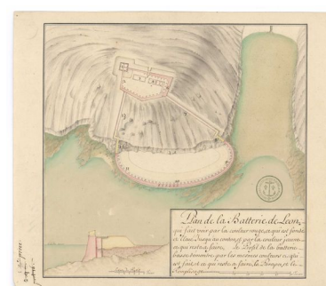
Plan de la batterie de Léon, fait en 1686 par Mollart. Plan général et profil des projets pour 1687 Repro. Service Historique de la Défense, Autr. Paul-Louis Mollart IVR53_20082908838NUCA
