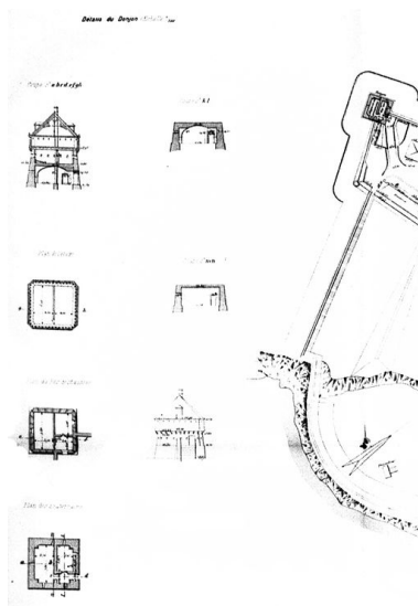
Plans et coupes de la tour d'artillerie du fort du Mengant, Direction d'Artillerie du génie de Brest, 10 août 1893, par le colonel Directeur d'Artillerie : Collomb Phot. Guillaume Lécueillier IVR53_20052903204NUCA
