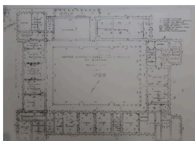
Centre d'apprentissage féminin de Quimper. Plan du rez-de-chaussée. Jacques Lachaud, architecte, 1953, 1958, 1960. Ce plan représente
