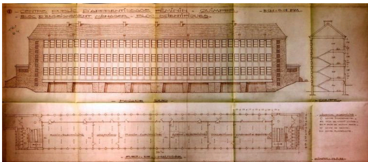
Élévation façade sud, coupe et plan du rez-de-chaussée. Centre public d'apprentissage féminin. Quimper. Bloc d'enseignement ménager. Bloc scientifique. Jacques Lachaud, architecte, 19/05/1962.
