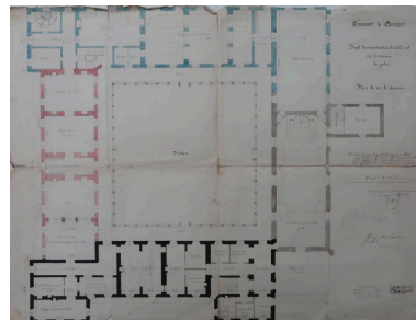
Plan du rez-de-chaussée, validé par le comité des inspecteurs généraux des édifices diocésains en 1860. Joseph Bigot, architecte. En noir, l'aile en cours de construction : différents parloirs, lingerie, salle d'étude, classe d'écritures saintes... en rouge et bleue, les ailes projetées. L'aile en bleue ne sera reconstruite qu'ultérieurement par l'architecte Henri Rapine.
