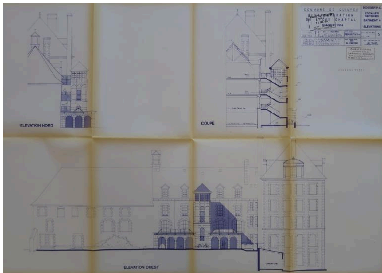
Escalier se secours, bâtiment A, élévations. Restructuration du lycée Chaptal, tranche 1994. Plan de masse et situation. Jean Bodereau, architecte, plans de novembre 1993.
