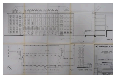
Extension d'un bâtiment pour l'aménagement du service de restauration. Façade ouest. État futur. Élévation, coupe,
