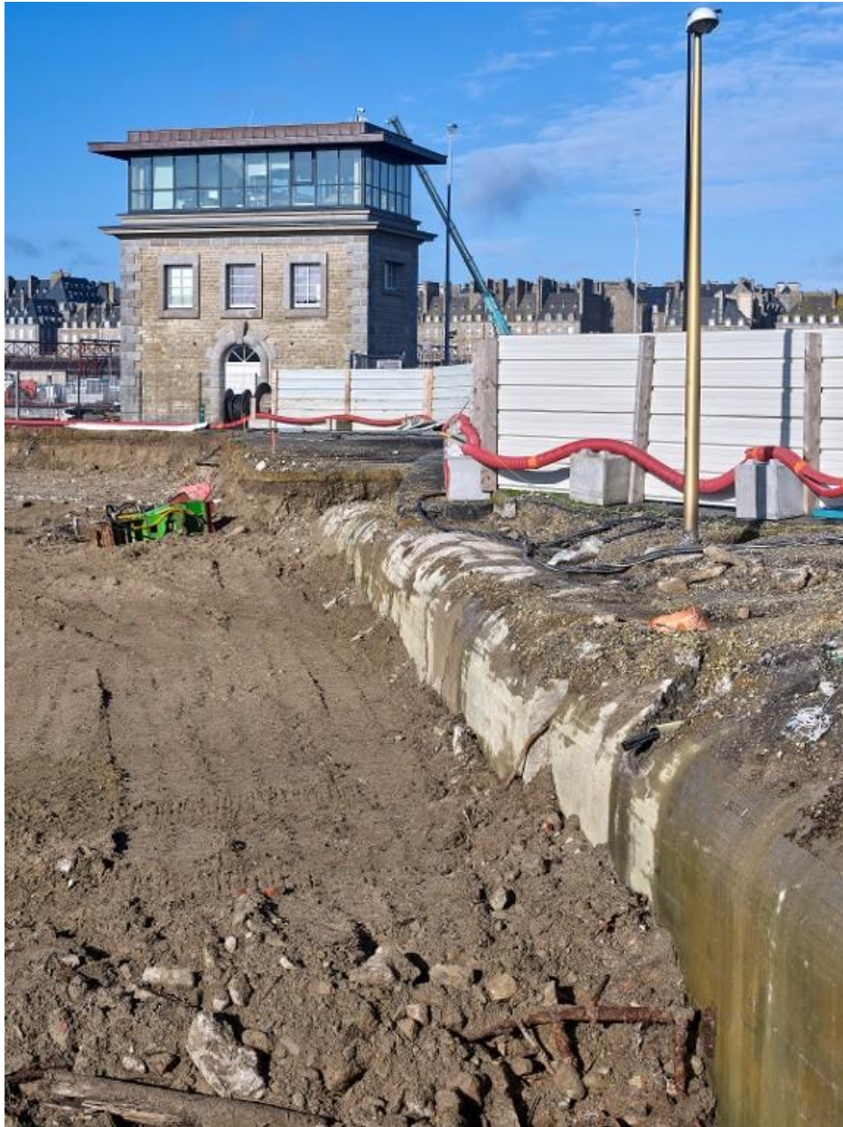
Vue de situation depuis le sud-est (couverture photographique du 22 janvier 2026). Sur la dalle de couverture du bunker passe la chaussée Éric Tabarly. En arrière-plan, le poste de commande de l'écluse du Naye
