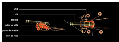
Reconstitution d'un canon sur son affût de marine par Art Graphique et Patrimoine (2001) Autr. Art Graphique et Patrimoine IVR53_20043511581NUCA
