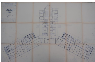
Bâtiment C Internat, plan du 1er étage. Réaménagement en internat du collège municipal, externat, internat et infirmerie, reconstruit après guerre. Noter les extensions des ailes pour satisfaire aux besoins de l'hygiène moderne. Albert Hec et Roger Besnard, architectes, 1966. Autr. Albert Hec, Autr. Roger Besnard IVR53_20203505067A1
