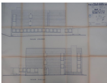
Bâtiment A, Administration Externat, Façades nord-est et sud-ouest. Noter le changement d'élévation de l'administration suite au déplacement des logements et le auvent de l'administration. Albert Hec et Roger Besnard, architectes, 1966.
