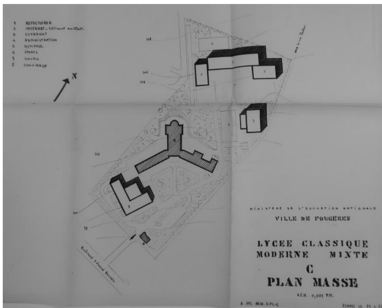
Plan masse du lycée classique et moderne mixte. Albert Hec, architecte, 1964.
