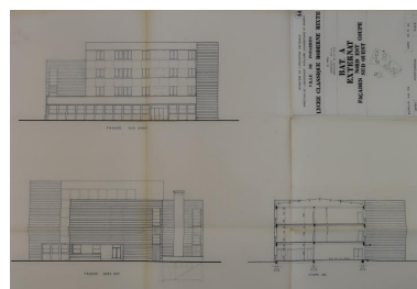
Bâtiment A Externat. Façades nord-ouest sud-est - Coupe. Projet non réalisé tel quel, Albert Hec, architecte, 1964. Autr. Albert Hec IVR53_20203505055A1
