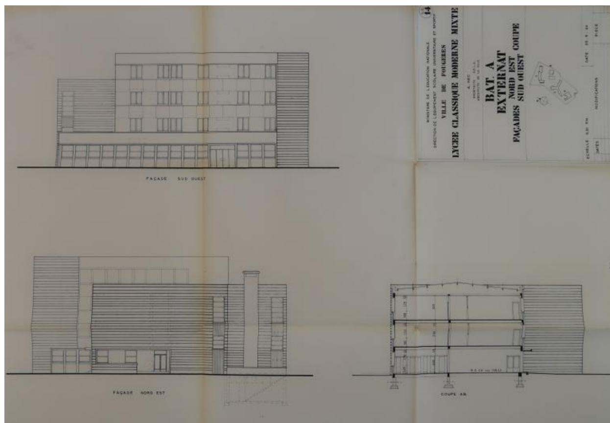
Bâtiment A Externat. Façades nord-ouest sud-est - Coupe. Projet non réalisé tel quel, Albert Hec, architecte, 1964.
