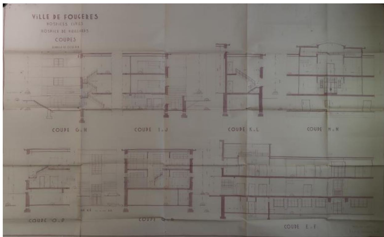
Bâtiment C Internat, ancien hospice de vieillards. Coupes. Albert Hec, architecte, 1936.
