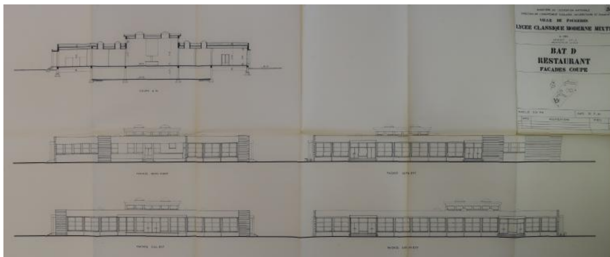
Bâtiment D Restaurant. Façades - Coupe. Albert Hec, architecte, 1964.
