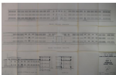
Bâtiment C Internat. Façades - Coupes. Albert Hec, architecte, 1964. Autr. Albert Hec IVR53_20203505056A0
