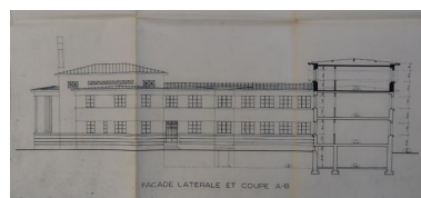
Bâtiment C Internat. Façades - Coupes : détail Façade latérale et coupe AB. Albert Hec, architecte, 1964. Autr. Albert Hec IVR53_20203505057A2
