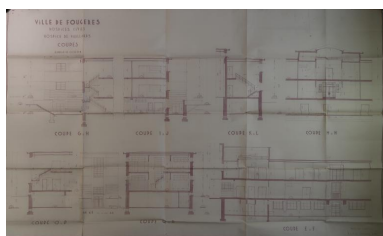
Bâtiment C Internat, ancien hospice de vieillards. Coupes. Albert Hec, architecte, 1936. Autr. Albert Hec IVR53_20203505049A0
