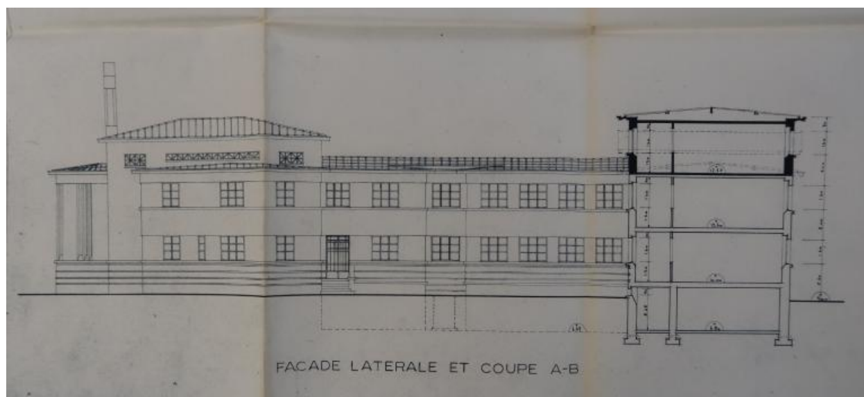
Bâtiment C Internat. Façades - Coupes : détail Façade latérale et coupe AB. Albert Hec, architecte, 1964.
