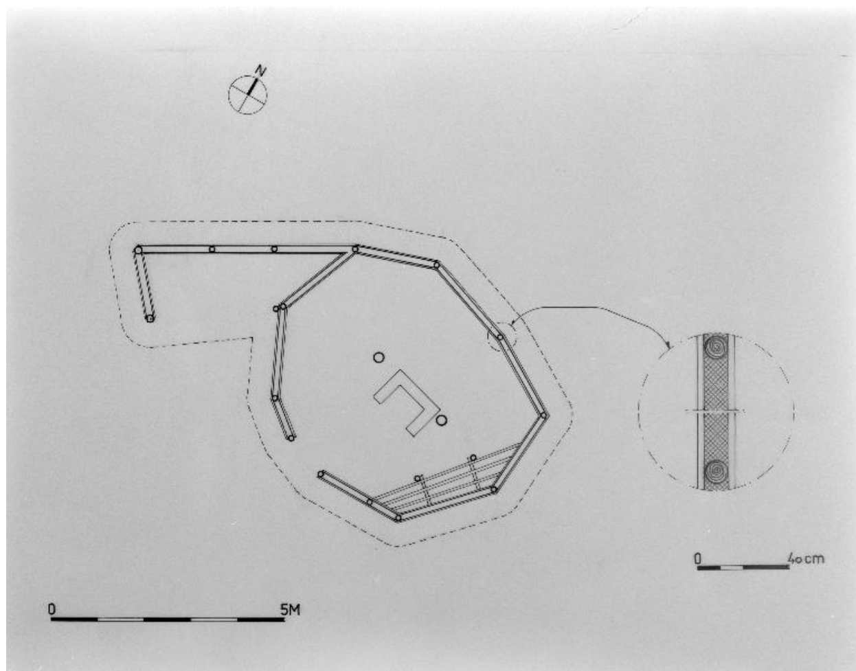
Plan au sol hutte de sabotier.
