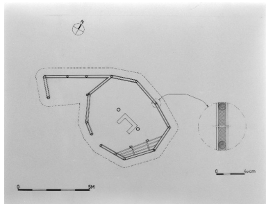
Plan au sol hutte de sabotier. Phot. Bernard Bègne, Autr. Yves Carpentier, Autr. Nicole Le Net IVR53_19995600525X
