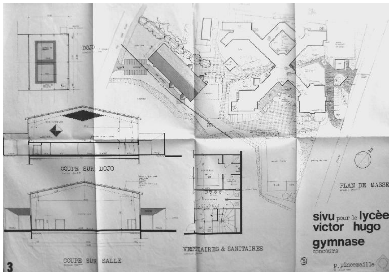
Plan de masse et coupes
