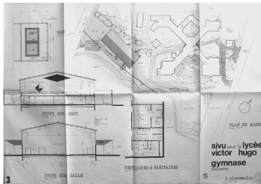
Plan de masse et coupes Phot. Philippe Bonnet IVR53_20185605026NUCA
