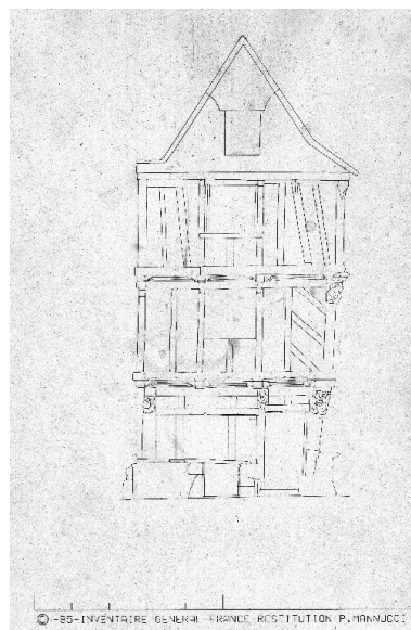
Photogrammétrie de l'élévation ouest (état en 1985) Phot. Norbert Lambart, Autr. Philippe Mannucci IVR53_19855600884P
