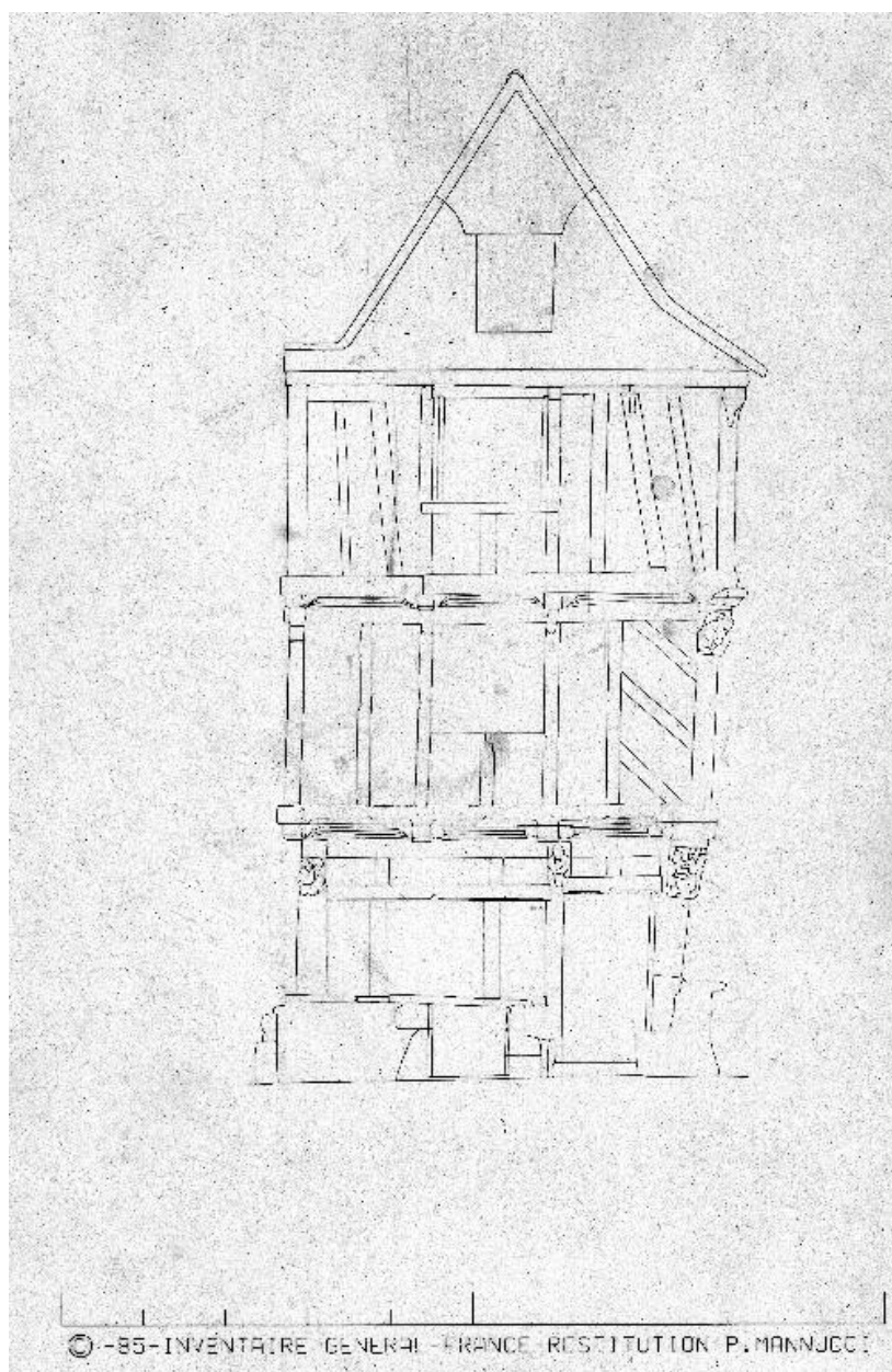
Photogrammétrie de l'élévation ouest (état en 1985)
