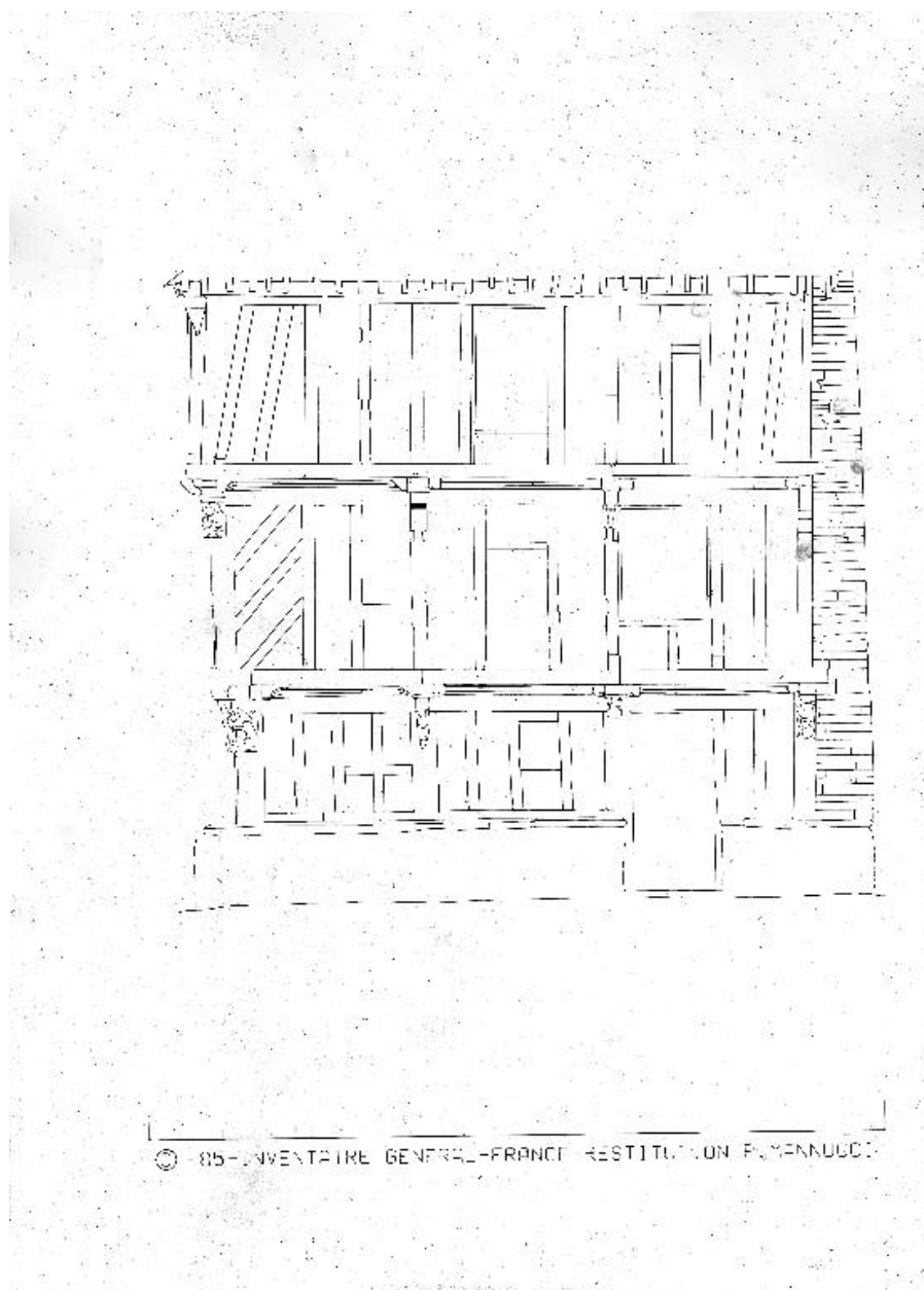
Photogrammétrie de l'élévation sud (état en 1985)
