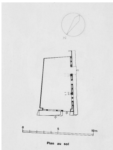
Plan au sol du rez-de-chaussée (état en 1985) Phot. Norbert Lambart, Autr. Philippe Boutroux IVR53_19855600586P
