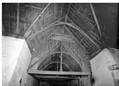
Vue de la charpente de la nef Phot. Guy Artur IVR53_19682201082V
