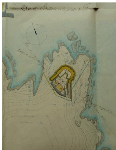
1 VH 294. Place de Belle-Ile, feuille n° 13 des projets extraordinaires pour 1857-1858, batterie de la pointe de Ramonet et détails des modifications apportées aux corps-de-garde types, 19 février 1857.
