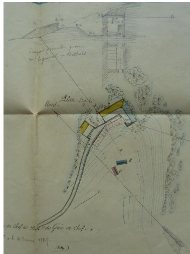
1 VH 292. Place de Belle-Ile, feuille n° 15 des projets extraordinaires pour 1847, établissement d'une batterie à Ramonet, 14 janvier 1847.
