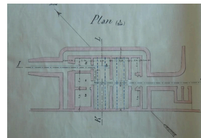
7 N 1904. Croquis joint au procès-verbal de conférence en date du 30 décembre 1894 relatif à l'emmagasinement des munitions dans les batteries de côte de Belle-Ile. Phot. Patrick Jadé IVR53_20175607371NUCA
