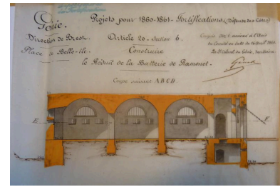
1 VK 534. Croquis n° 1 annexé à l'avis du Comité en date du 16 avril 1861, construire le réduit de la batterie de Ramonnet. Phot. Patrick Jadé IVR53_20175607357NUCA
