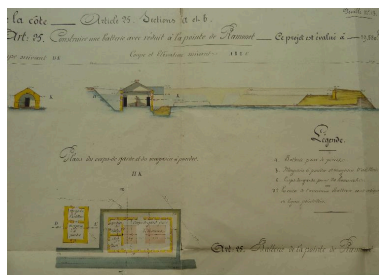
1 VH 294. Place de Belle-Ile, feuille n° 13 des projets extraordinaires pour 1857-1858, batterie de la pointe de Ramonet et détails des modifications apportées aux corps-de-garde types, 19 février 1857.
