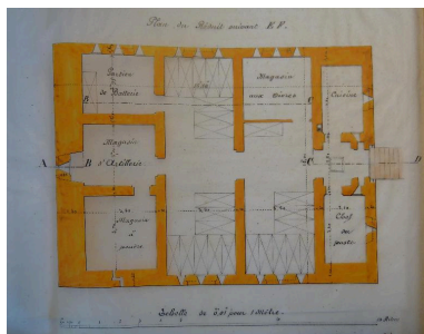
1 VK 534. Croquis n° 1 annexé à l'avis du Comité en date du 16 avril 1861, construire le réduit de la batterie de Ramonnet. Phot. Patrick Jadé IVR53_20175607358NUCA
