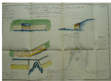
1 VH 292. Place de Belle-Île, feuille n° 15 des projets extraordinaires pour 1847, établissement d'une batterie à Ramonet, 14 janvier 1847.
