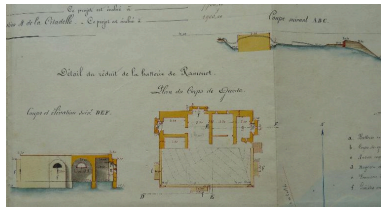
1 VH 296. Place de Belle-Ile, feuille n° 11 des projets supplémentaires pour 1860-1861, batterie de Ramonnet, batterie du Vésuve, bastion 4 de la citadelle, 24 novembre 1860. Phot. Patrick Jadé IVR53_20175607355NUCA
