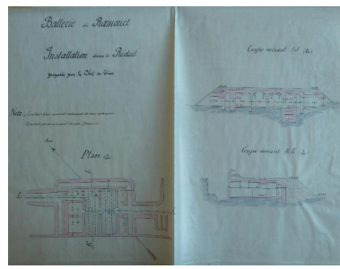
7 N 1904. Croquis joint au procès-verbal de conférence en date du 30 décembre 1894 relatif à l'emmagasinement des munitions dans les batteries de côte de Belle-Ile. Phot. Patrick Jadé IVR53_20175607370NUCA
