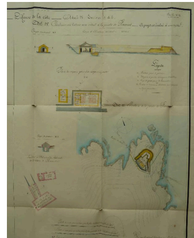
1 VH 294. Place de Belle-Ile, feuille n° 13 des projets extraordinaires pour 1857-1858, batterie de la pointe de Ramonet et détails des modifications apportées aux corps-de-garde types, 19 février 1857.
