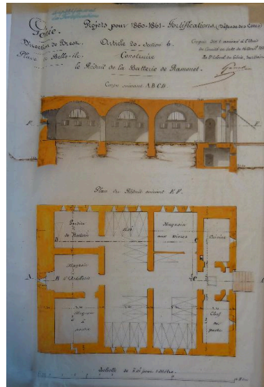
1 VK 534. Croquis n° 1 annexé à l'avis du Comité en date du 16 avril 1861, construire le réduit de la batterie de Ramonnet. Phot. Patrick Jadé IVR53_20175607356NUCA
