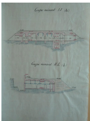
7 N 1904. Croquis joint au procès-verbal de conférence en date du 30 décembre 1894 relatif à
