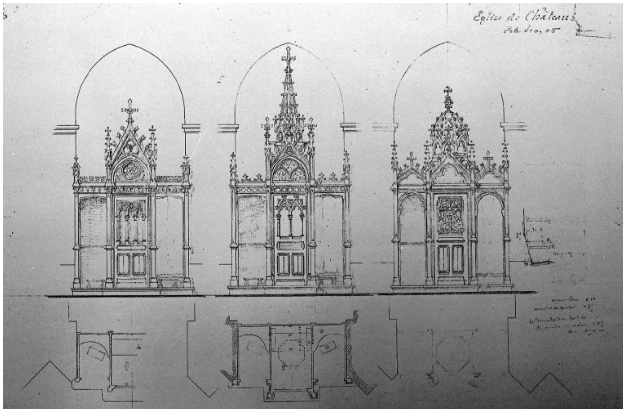
Elévations des confessionnaux.
