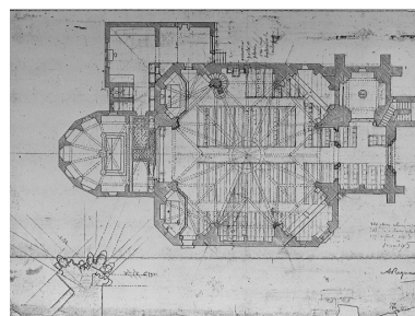
Plan de l'église : projet. L'ancienne porte a été placée sur une façade latérale. Phot. Guy Artur, Phot. Norbert Lambart, Autr. Arthur Regnault IVR53_19973500171X
