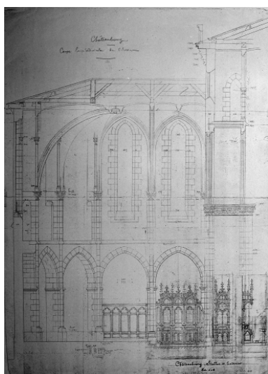
Coupe du choeur : stalles et boiseries. Phot. Guy Artur, Phot. Norbert Lambart, Autr. Arthur Regnault IVR53_19973500172X
