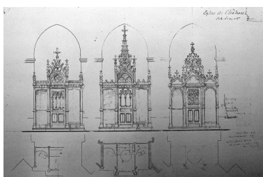
Elévations des confessionnaux. Phot. Guy Artur, Phot. Norbert Lambart, Autr. Arthur Regnault IVR53_19973500173X
