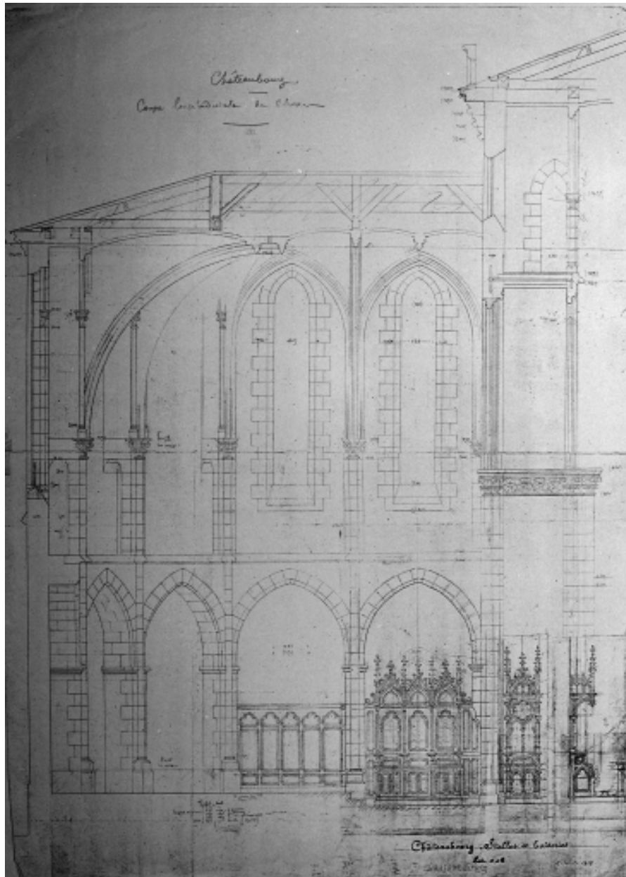
Coupe du chœur : stalles et boiseries.
