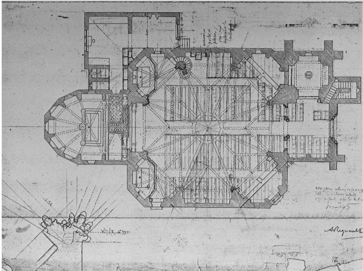
Plan de l'église : projet. L'ancienne porte a été placée sur une façade latérale.
