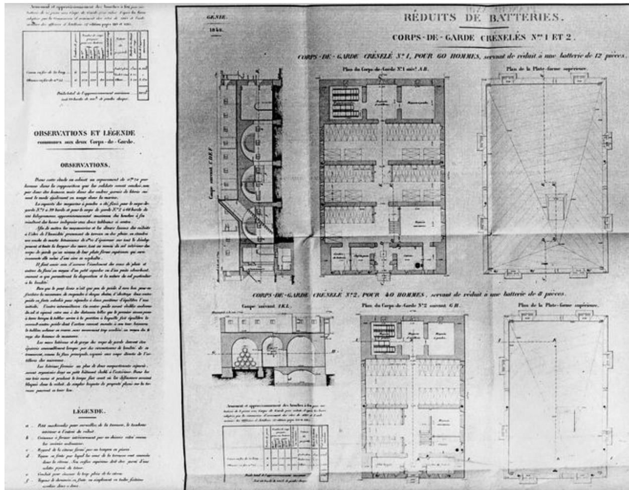
Plans, coupes et profils des réduits de batteries : corps de garde crénelés n° 1 (pour 60 hommes, servant de réduit à une batterie de 12 pièces) et n° 2 (pour 40 hommes, servant de réduit à une batterie de 8 pièces), 1846
