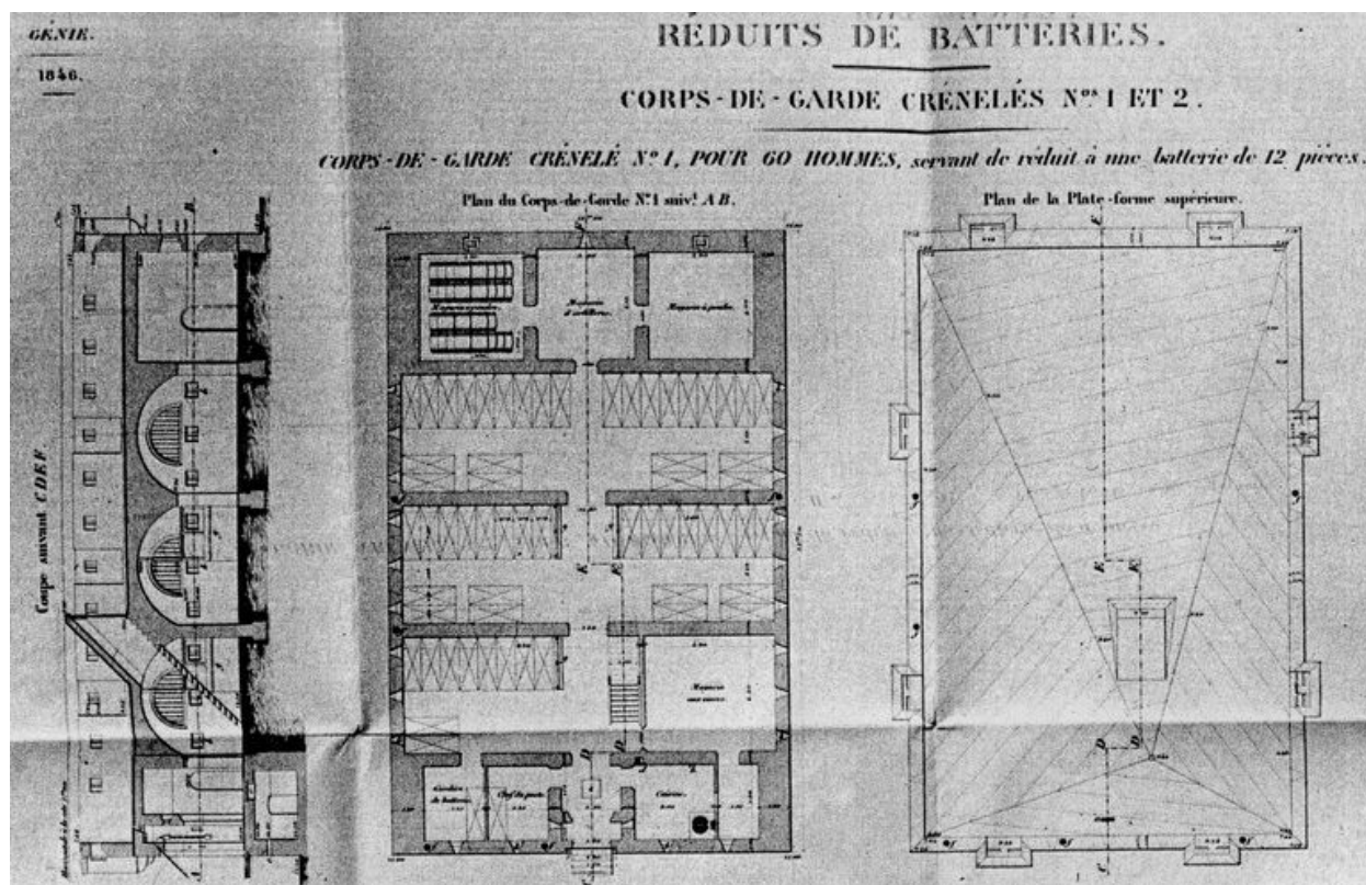
Plans, coupes et profils des réduits de batteries : corps de garde crénelés n° 1 et 2, 1846, détail du corps de garde crénelés n° 1 pour 60 hommes, servant de réduit à une batterie de 12 pièces
