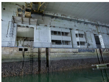
Vue de l'alvéole D : quai ouest n° 20. Dans l'épaisseur du mur de refend entre les alvéoles C et D se trouvent les salles des pompes d'épuisement et d'assèchement Phot. Bernard Bègne IVR53_20215600510NUCA
