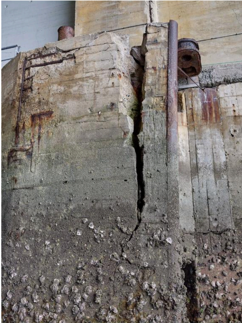
Vue de l'entrée de l'alcôve D : entrée du quai n° 19 est montrant le vieillissement du béton armé
