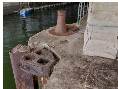
Vue de l'entrée de l'alvéole D : quai est n° 19 avec cabestan, fixation haute de la porte d'écluse. Elle est maintenue par deux tiges filetées de réglage noyées dans le béton Phot. Bernard Bègne IVR53_20235600099NUCA
