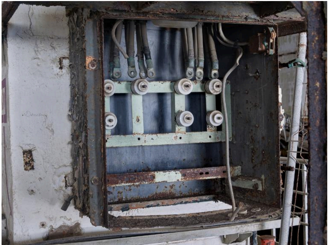
Vue du mur de refend situé entre les alvéoles C et D : tableau situé sous l'armoire électrique
