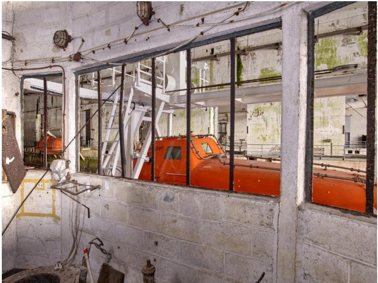
Vue de la salle des pompes située entre les alvéoles D (n° 19, 19a et 20) et E (n° 17 et 18)
