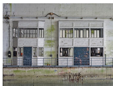
Vue générale des salles des pompes aménagées dans l'épaisseur du mur de refend entre les alvéoles D et E. Au premier plan, le quai n° 19 Phot. Bernard Bègne IVR53_20235600110NUCA
