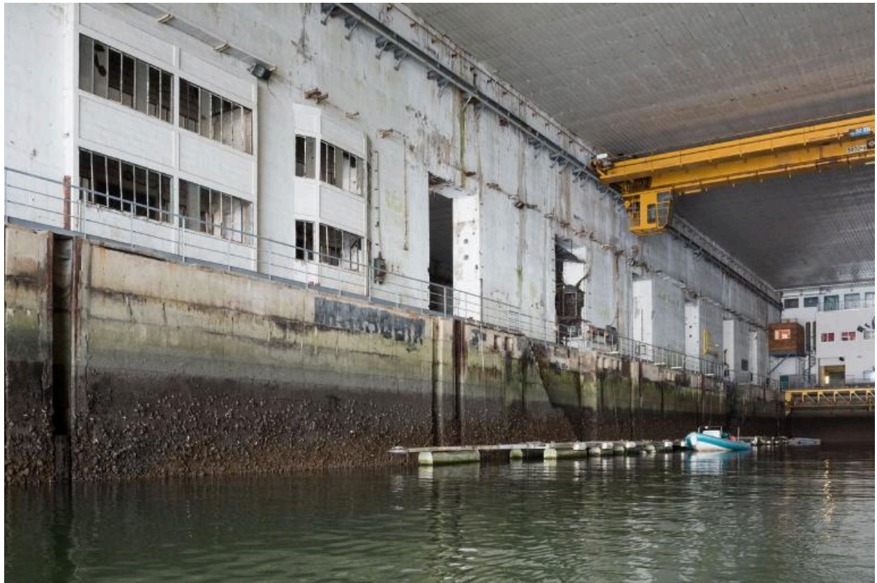
Vue de l'alcôve D en eau : quai n° 20 et salles des pompes aménagées dans l'épaisseur du mur de refend entre les alcôves C et D
