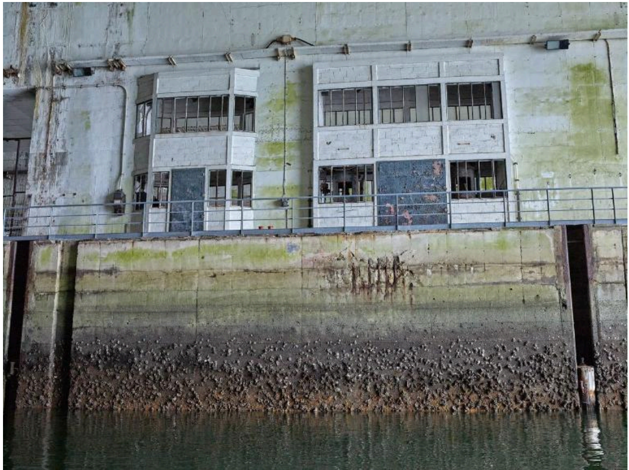
Vue de l'algéole D : quai est (quai n° 19). Dans l'épaisseur du mur de refend entre les algéoles D et E se trouvent les salles des pompes d'épuisement et d'assèchement
