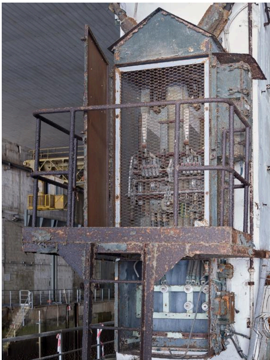
Vue du mur de refend situé entre les alvéoles C et D : armoire électrique
