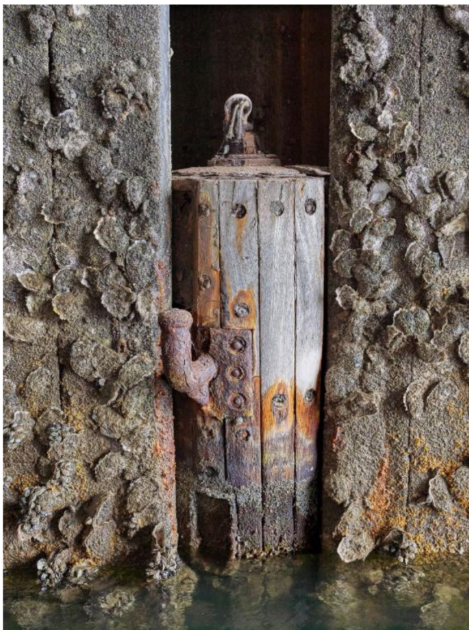
Vue de l'alvéole D : quai est n° 19, dispositif flottant amarrage suivant la hauteur d'eau
