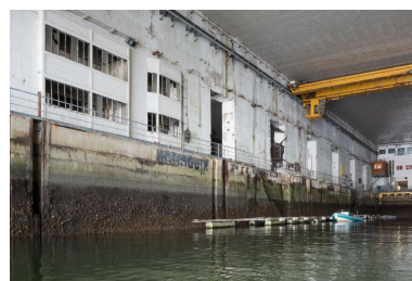
Vue de l'alvéole D en eau : quai n° 20 et salles des pompes aménagées dans l'épaisseur du mur de refend entre les alvéoles C et D Phot. Charlotte Barraud IVR53_20215600606NUCA
