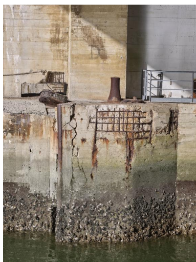
Vue de l'entrée de l'alvéole : quai ouest n° 20 avec cabestan. A signaler : la fixation haute de la
