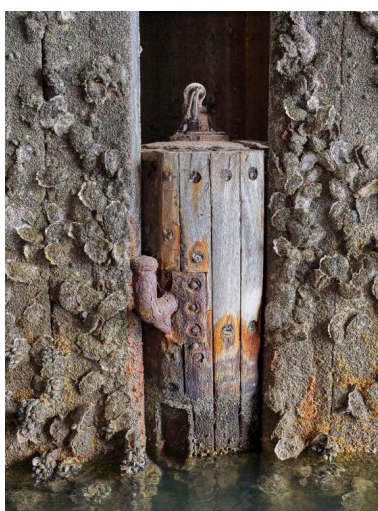
Vue de l'alvéole D : quai est n° 19, dispositif flottant amarrage suivant la hauteur d'eau Phot. Bernard Bègne IVR53_20215600513NUCA
