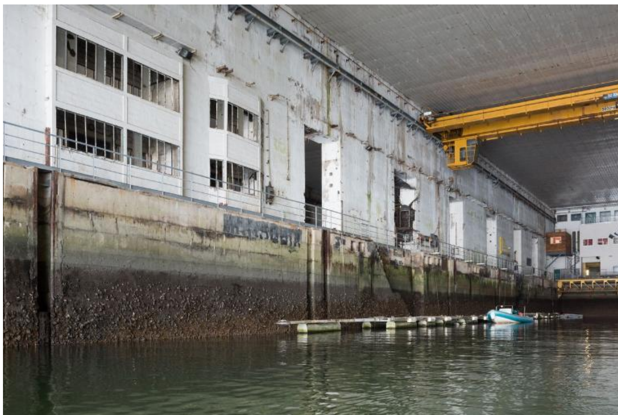
Vue de l'algéole D en eau : quai n° 20 et salles des pompes aménagées dans l'épaisseur du mur de refend entre les algéoles C et D
