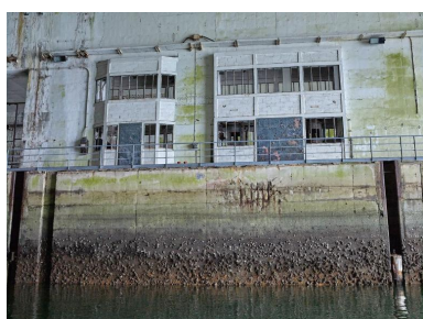
Vue de l'alvéole D : quai est (quai n° 19). Dans l'épaisseur du mur de refend entre les alvéoles D et E se trouvent les salles des pompes d'épuisement et d'assèchement Phot. Bernard Bègne IVR53_20215600512NUCA
