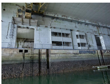
Vue de l'alvéole D : quai ouest n° 20. Dans l'épaisseur du mur de refend entre les alvéoles C et D se trouvent les salles des pompes d'épuisement et d'assèchement Phot. Bernard Bègne IVR53_20215600510NUCA
