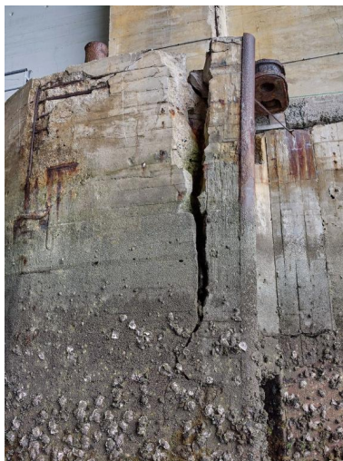
Vue de l'entrée de l'alvéole D : entrée du quai n° 19 est montrant le vieillissement du béton armé Phot. Bernard Bègne IVR53_20215600515NUCA
