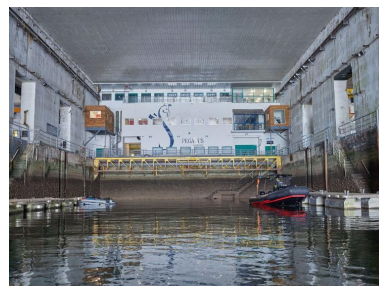
Vue de l'alvéole D (n° 19, 19a et 20) en eau. Au fond de cette alvéole, dans les ateliers, est installée l'entreprise Pegasus Leadership Phot. Bernard Bègne IVR53_20215600511NUCA
