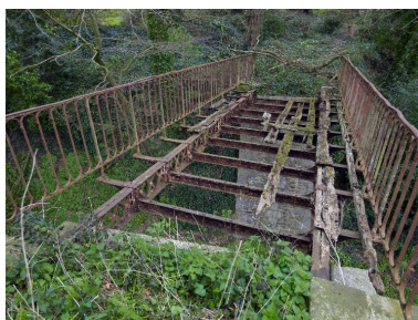
Passerelle métallique. Vue générale du tablier Phot. Bernard Bègne IVR53_20152200431NUCA
