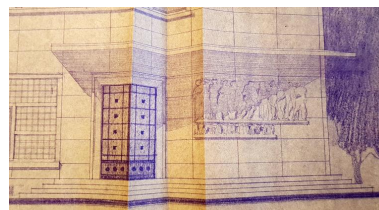
Internat : détail d'une élévation de la façade sud, non exécuté (G. Tourry architecte chef de groupe, Baudeau, Conan, Grihangne, architectes, janvier 1952) Dess. Georges Tourry, Dess. Henri Conan, Dess. Baudeau, Dess. René Grihangne IVR53_20185606671A1
