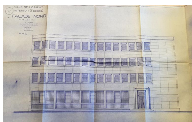
Internat : élévation de la façade nord (G. Tourry architecte chef de groupe, Baudeau, Conan, Grihangne, architectes, 20/01/1953). Dess. Georges Tourry, Dess. Henri Conan, Dess. Baudeau, Dess. René Grihangne IVR53_20185606672A1
