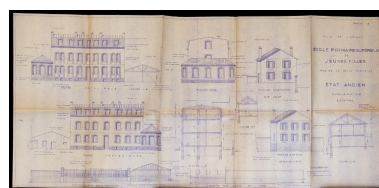
Élévations et coupes de l'école primaire supérieure de jeunes filles de Lorient, détruite pendant la Seconde Guerre mondiale, dressées par l'architecte R. Grihaigne, afin de chiffrer les dommages de guerre. Phot. Bernard Bègne IVR53_20205600474NUCA
