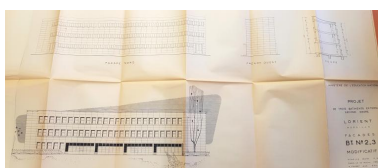
Elévation d'une façade d'un bâtiment d'externat (G. Tourry, architecte, 10/02/1954) Dess. Georges Tourry IVR53_20185606676A1
