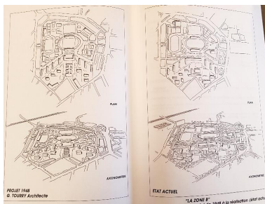
Comparaison du plan masse d'origine et plan masse réalisé. Autr. Atelier de l'Ile IVR53_20185606505NUCA
