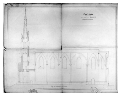
Coupe longitudinale (Projet du 13/11/1851) Repro. François Dagorn IVR53_19683500308V
