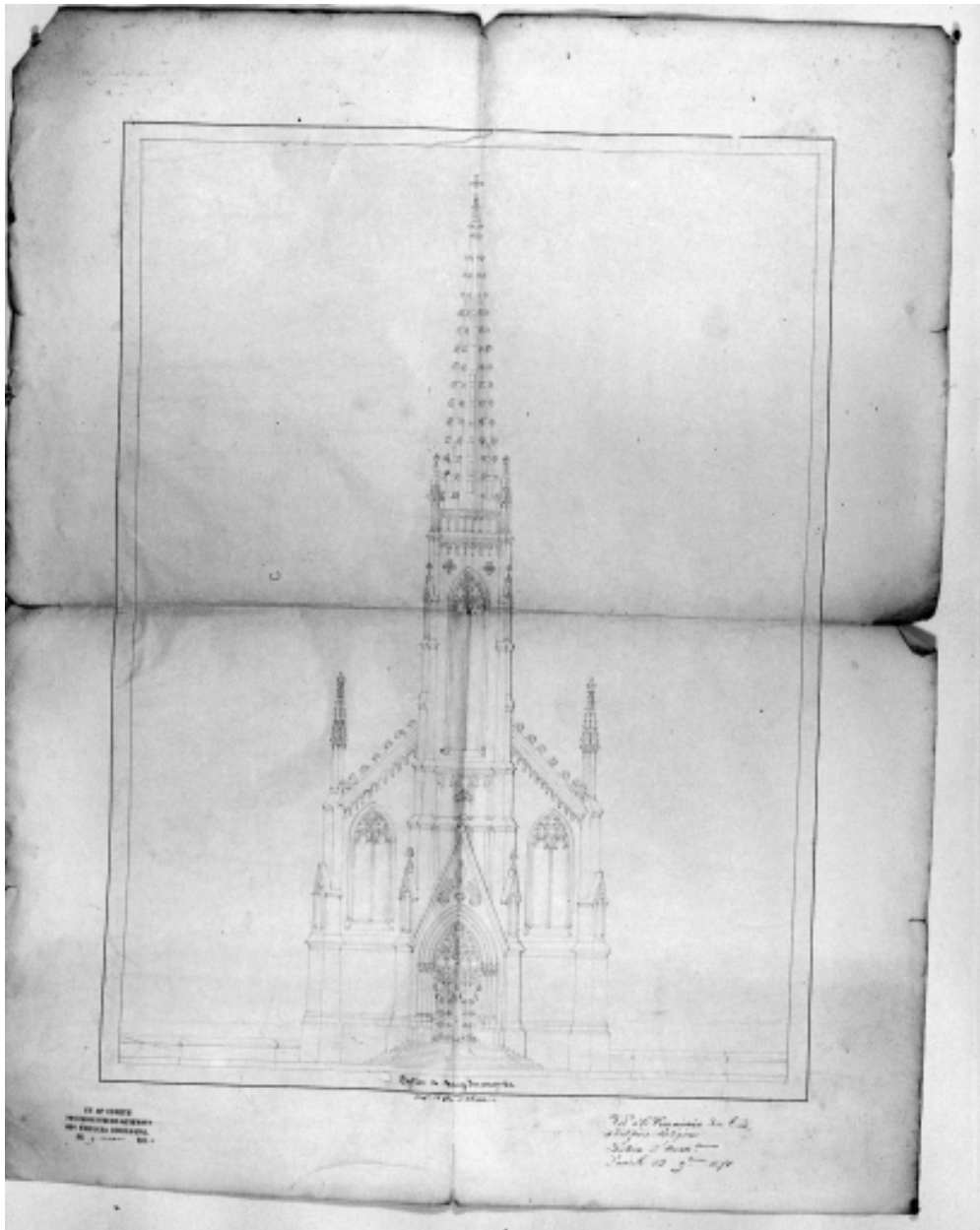
Elévation Ouest (Projet du 13/11/1851)
