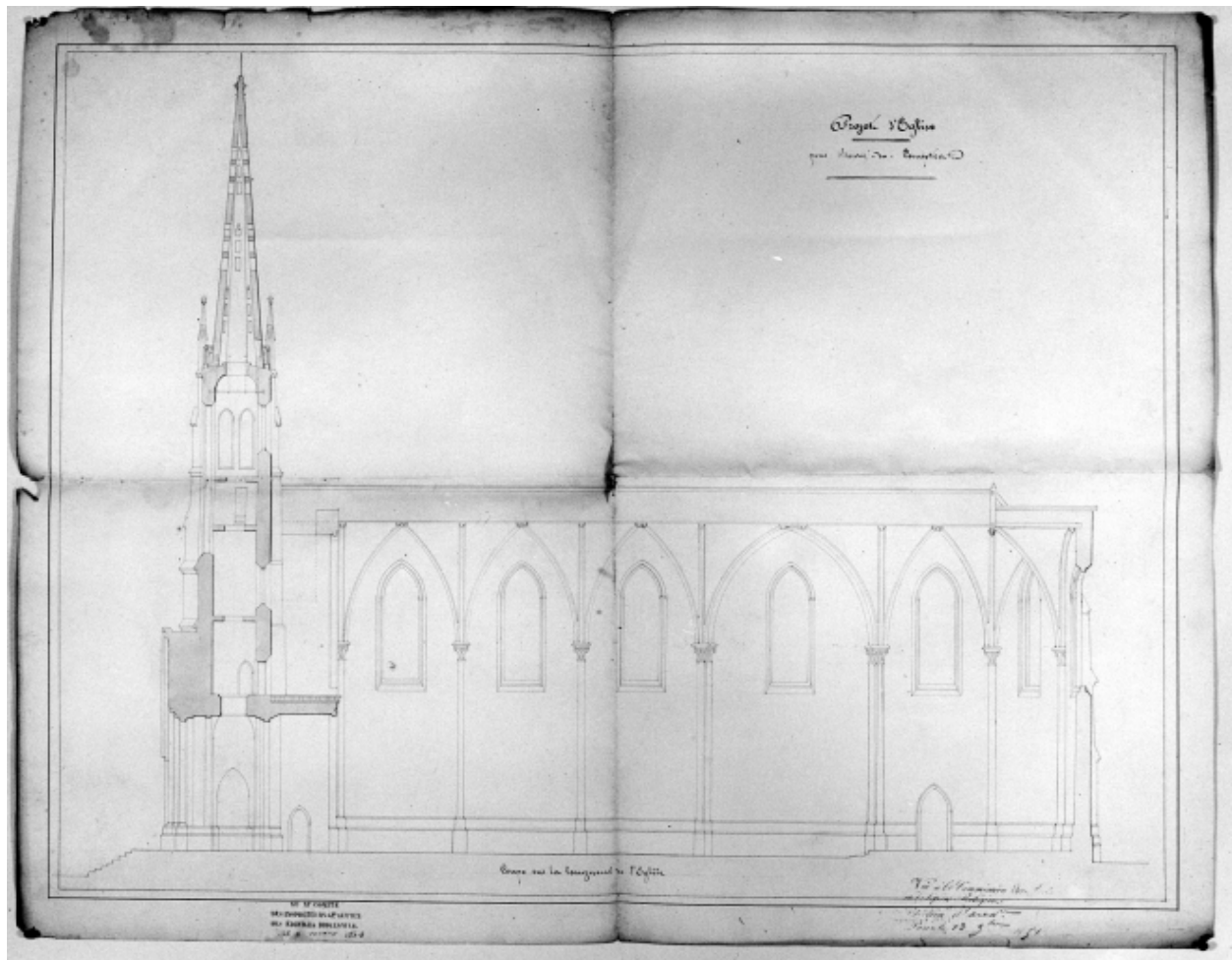
Coupe longitudinale (Projet du 13/11/1851)
