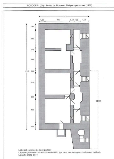
Plan du bunker - abri de type 661 SK (dessin : Olivier Dohér, 1982) Phot. Olivier Dohér IVR53_20232905365NUCA
