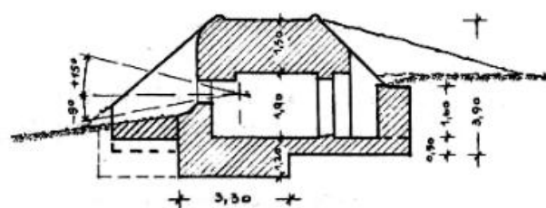
Schnitt A-B
