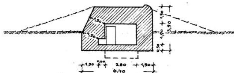
Schnitt C-D
