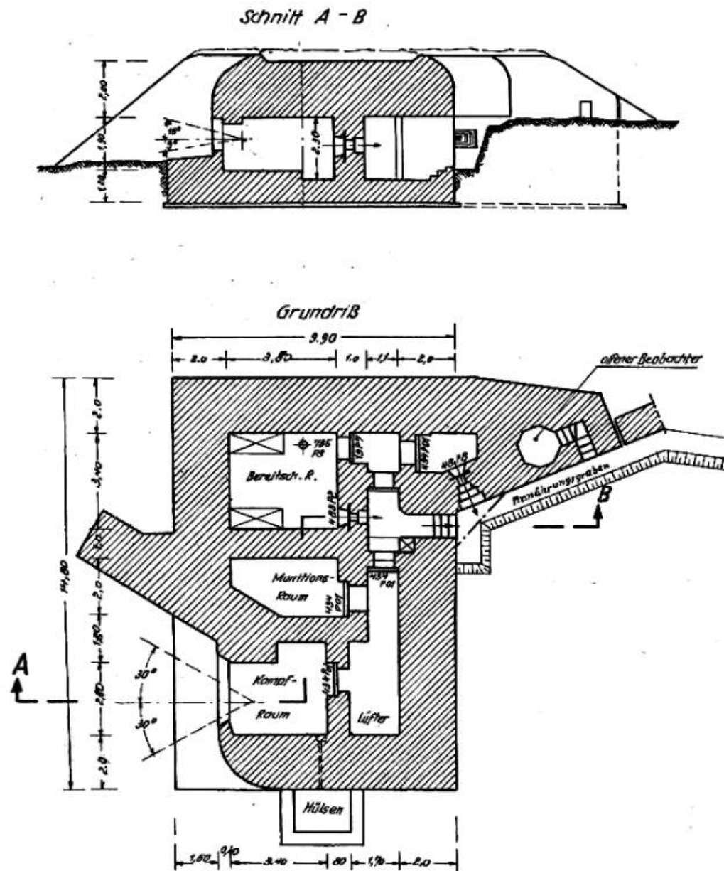
Plan-type d'un bunker de type 653 pour un canon antchar de 5 cm (Schartenstand für 5 cm KwK)
