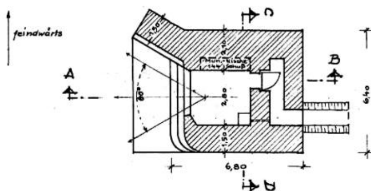
Grundriß
