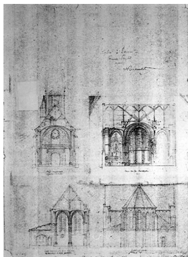
Coupe de l'église Repro. Guy Artur, Repro. Norbert Lambart IVR53_19973500133XB
