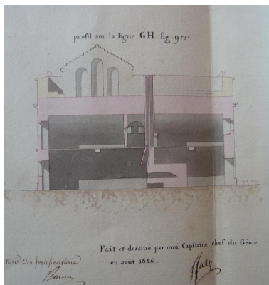
1 VH 1516. Direction du Génie de Port-Louis, Poste de Quiberon, feuille n° 2 des projets pour 1827, profils de la caserne défensive du fort Penthièvre, août 1826. Phot. Patrick Jadé IVR53_20175607108NUCA
