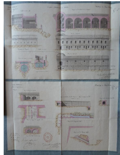
1 VH 1515. Direction du Génie de Port-Liberté, Poste de Quiberon, an 11 [1802-1803], élévations, coupes et plans de la caserne, des casemates à feux de revers, du corps de garde à construire au fort Penthièvre d'après la décision du ministre du 21 ventôse an 11 [13 mars 1803].
