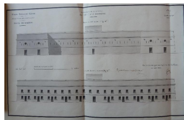
1 VH 1516. Direction du Génie de Port-Louis, Poste de Quiberon, feuille n° 3 des projets pour 1827, élévation de la caserne défensive du fort Penthièvre, août 1826. Phot. Patrick Jadé IVR53_20175607098NUCA
