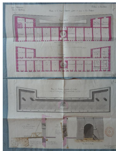
1 VH 1515. Direction du Génie de Port-Liberté, Poste de Quiberon, an 11 [1802-1803], plans de la caserne défensive projetée à la gorge du fort Penthievre, prairial an 11 [mai-juin 1803].
