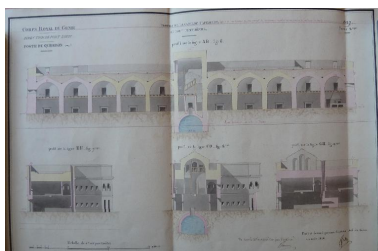
1 VH 1516. Direction du Génie de Port-Louis, Poste de Quiberon, feuille n° 2 des projets pour 1827, profils de la caserne défensive du fort Penthièvre, août 1826. Phot. Patrick Jadé IVR53_20175607105NUCA
