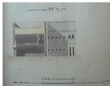
1 VH 1516. Direction du Génie de Port-Louis, Poste de Quiberon, feuille n° 2 des projets pour 1827, profils de la caserne défensive du fort Penthièvre, août 1826. Phot. Patrick Jadé IVR53_20175607106NUCA
