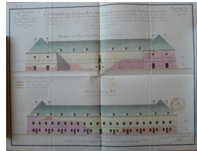
1 VH 1515. Direction du Génie de Port-Liberté, Travaux extraordinaires du fort Penthievre, élévations de la caserne en construction à la gorge du fort Penthievre, servant à faire connaître sa situation au 30 décembre 1808. Phot. Patrick Jadé IVR53_20175607093NUCA
