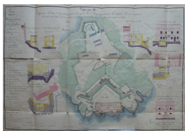
1 VH 1516. Direction du Génie de Nantes, Place de Quiberon, feuille des projets pour 1834, plan général du fort Penthievre et de son camp retranché, 25 mars 1834. Phot. Patrick Jadé IVR53_20175607121NUCA
