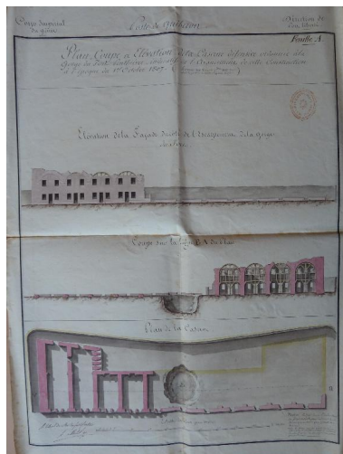
1 VH 1515. Direction du Génie de Port-Liberté, Poste de Quiberon, plan, coupe et élévation de la caserne défensive ordonnée à la gorge du fort Penthièvre, indicatifs de l'avancement de cette construction à l'époque du 1er octobre 1807.
