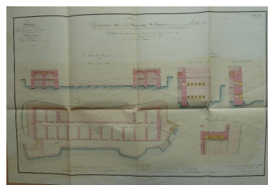
1 VH 1517. Direction du Génie de Nantes, Place de Quiberon, feuille n° 2 des projets pour 1844, modifier l'ouverture extérieure des créneaux de la caserne A, 1er février 1844. Phot. Patrick Jadé IVR53_20175607109NUCA
