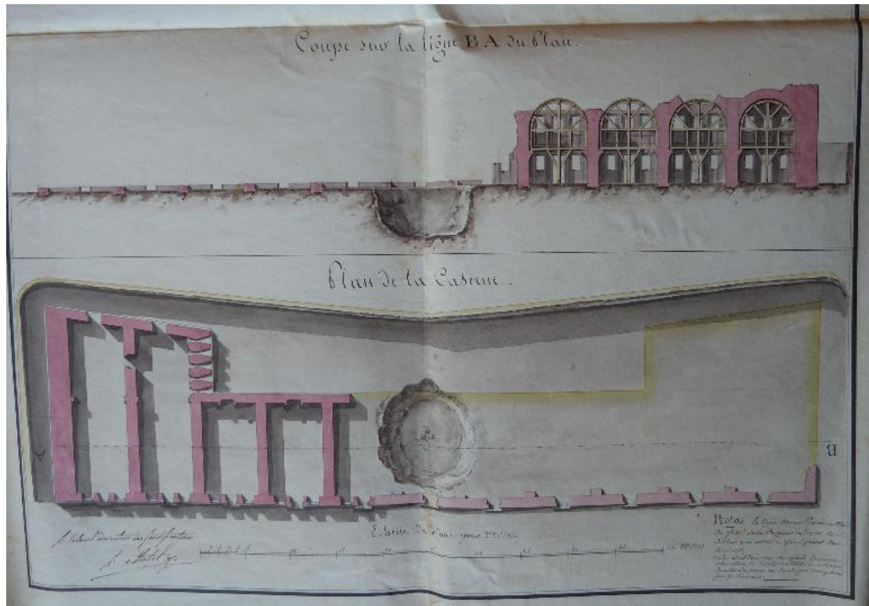
1 VH 1515. Direction du Génie de Port-Liberté, Poste de Quiberon, plan, coupe et élévation de la caserne défensive ordonnée à la gorge du fort Penthievre, indicatifs de l'avancement de cette construction à l'époque du 1er octobre 1807.
