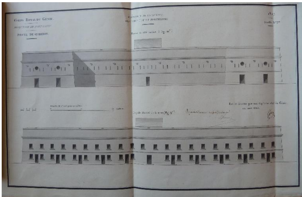
1 VH 1516. Direction du Génie de Port-Louis, Poste de Quiberon, feuille n° 3 des projets pour 1827, élévation de la caserne défensive du fort Penthievre, août 1826.
