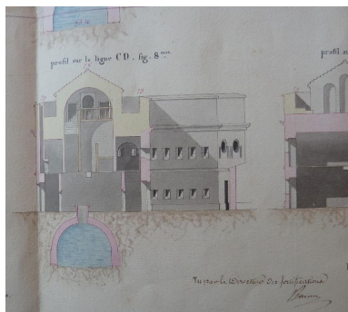
1 VH 1516. Direction du Génie de Port-Louis, Poste de Quiberon, feuille n° 2 des projets pour 1827, profils de la caserne défensive du fort Penthièvre, août 1826. Phot. Patrick Jadé IVR53_20175607107NUCA
