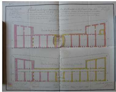
1 VH 1515. Direction du Génie de Port-Liberté, Travaux extraordinaires du fort Penthievre, plans du rez de chaussée et du premier étage de la caserne en construction à la gorge du fort Penthievre, servant à faire connaître sa situation au 30 décembre 1808. Phot. Patrick Jadé IVR53_20175607092NUCA
