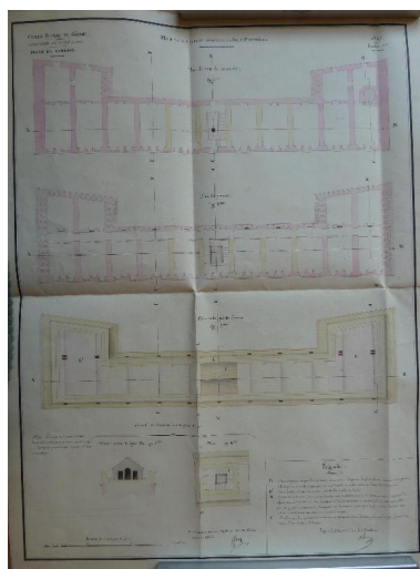
1 VH 1516. Direction du Génie de Port-Louis, Poste de Quiberon, feuille n° 1 des projets pour 1827, plan de la caserne défensive du fort Penthievre, août 1826.
