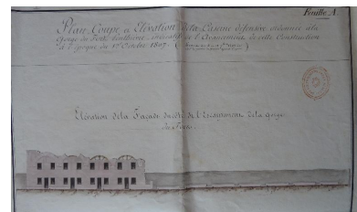
1 VH 1515. Direction du Génie de Port-Liberté, Poste de Quiberon, plan, coupe et élévation de la caserne défensive ordonnée à la gorge du fort Penthièvre, indicatifs de l'avancement de cette construction à l'époque du 1er octobre 1807.
