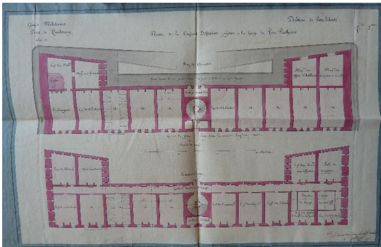
1 VH 1515. Direction du Génie de Port-Liberté, Poste de Quiberon, an 11 [1802-1803], plans de la caserne défensive projetée à la gorge du fort Penthievre, prairial an 11 [mai-juin 1803].
