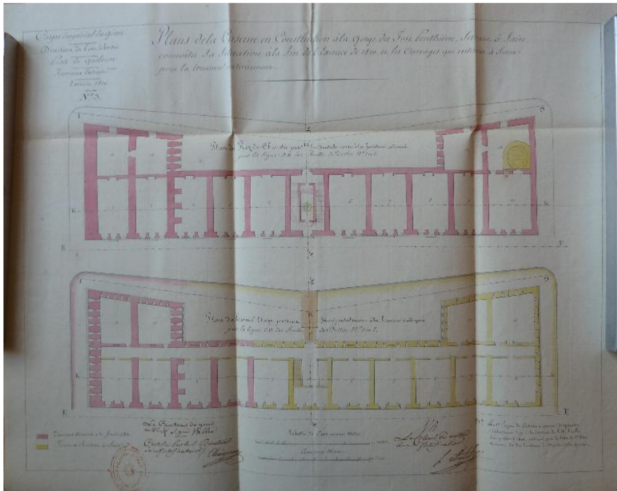
1 VH 1515. Direction du Génie de Port-Liberté, Poste de Quiberon, plans de la caserne en construction à la gorge du fort Penthièvre, servant à faire connaître sa situation à la fin de l'année de 1810.
