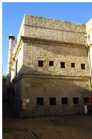
Saint-Pierre-Quiberon, fort de Penthievre, caserne défensive, flanc du demi-bastion sud-ouest. Phot. Lionel Duigou IVR53_20175606632NUCA
