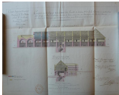
1 VH 1515. Direction du Génie de Port-Liberté, Poste de Quiberon, coupes de la caserne en construction à la gorge du fort Penthievre, servant à faire connaître sa situation à la fin de l'année de 1810. Phot. Patrick Jadé IVR53_20175607095NUCA
