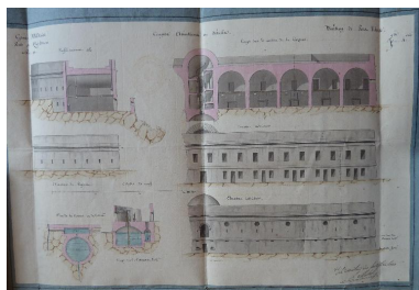
1 VH 1515. Direction du Génie de Port-Liberté, Poste de Quiberon, an 11 [1802-1803], élévations, coupes et plans de la caserne, des casemates à feux de revers, du corps de garde à construire au fort Penthièvre d'après la décision du ministre du 21 ventôse an 11 [13 mars 1803].
