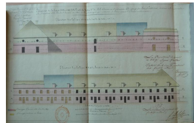
1 VH 1515. Direction du Génie de Port-Liberté, Poste de Quiberon, élévations de la caserne en construction à la gorge du fort Penthievre, servant à faire connaître sa situation à la fin de l'année de 1810. Phot. Patrick Jadé IVR53_20175607096NUCA
