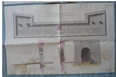
1 VH 1515. Direction du Génie de Port-Liberté, Poste de Quiberon, an 11 [1802-1803], plans de la caserne défensive projetée à la gorge du fort Penthièvre, prairial an 11 [mai-juin 1803].
