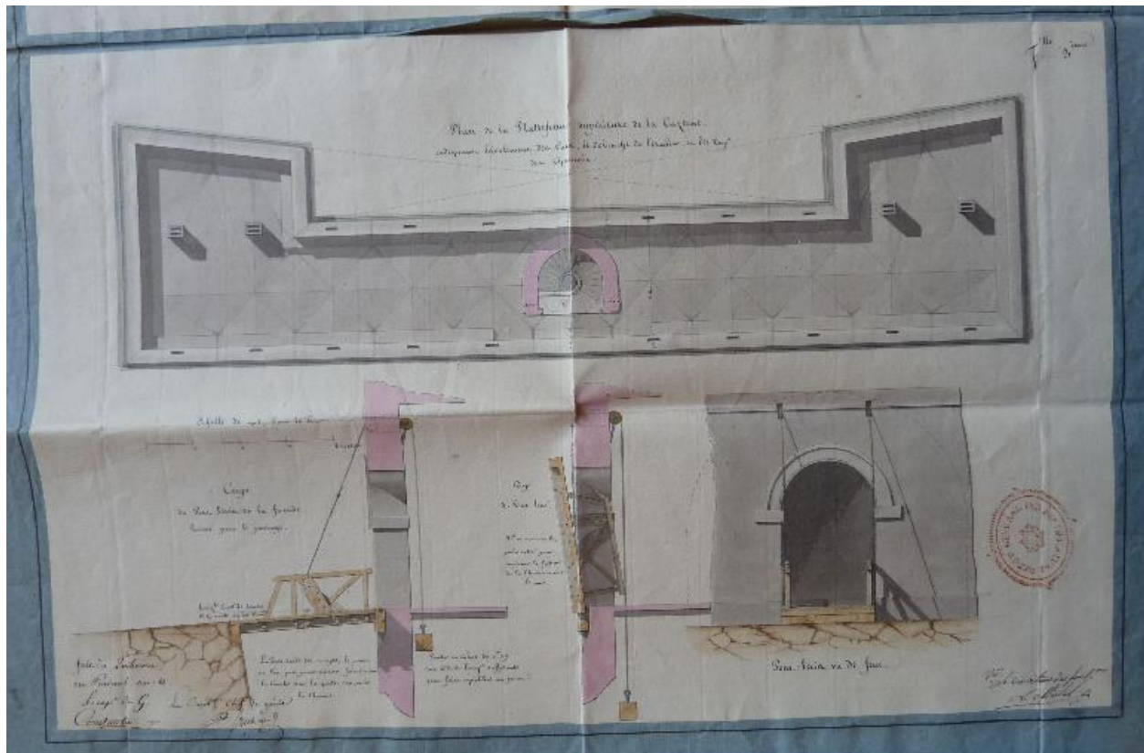
1 VH 1515. Direction du Génie de Port-Liberté, Poste de Quiberon, an 11 [1802-1803], plans de la caserne défensive projetée à la gorge du fort Penthievre, prairial an 11 [mai-juin 1803].
