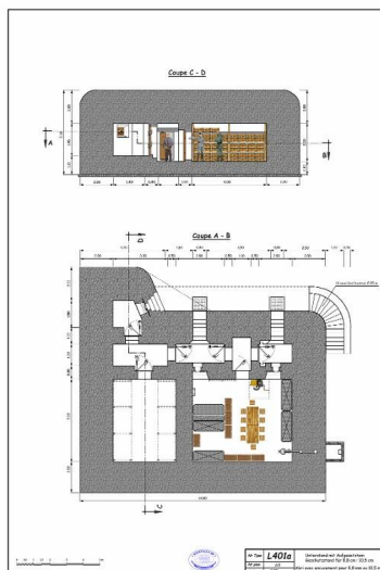
Plan et coupe d'un bunker-abri-magasin de munitions de type L 401a avec cuve pour canon antiaérien de 10,5 cm (Unterstand mit aufgesetztem Geschützstand für 8,8/10,5 cm Flak)
