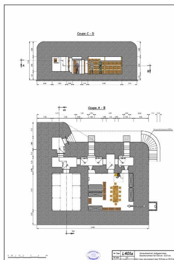
Plan et coupe d'un bunker-abri-magasin de munitions de type L 401a avec cuve pour canon antiaérien de 10,5 cm (Unterstand mit aufgesetztem Geschützstand für 8,8/10,5 cm Flak) Dess. Christian Moigneux IVR53_20263510107NUDA
