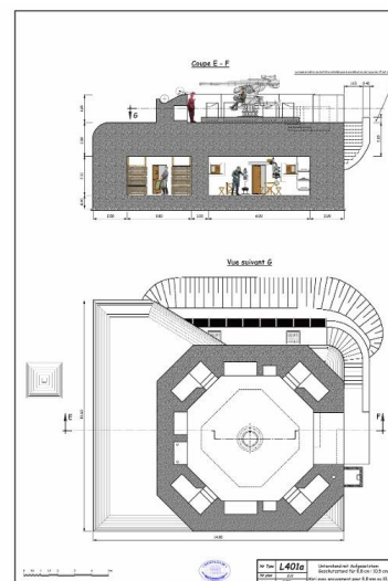
Plans et coupes d'un bunker-abri-magasin de munitions de type L 401a avec cuve pour canon antiaérien de 10,5 cm (Unterstand mit aufgesetztem Geschützstand für 8,8/10,5 cm Flak) Dess. Christian Moigneux IVR53_20263510108NUDA
