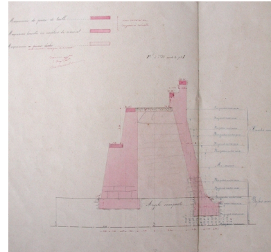
Projet de parapet sur la grande jetée en 1848 (AD 22) Repro. Guy Prigent, Phot. Tessier IVR53_20072207750NUCB
