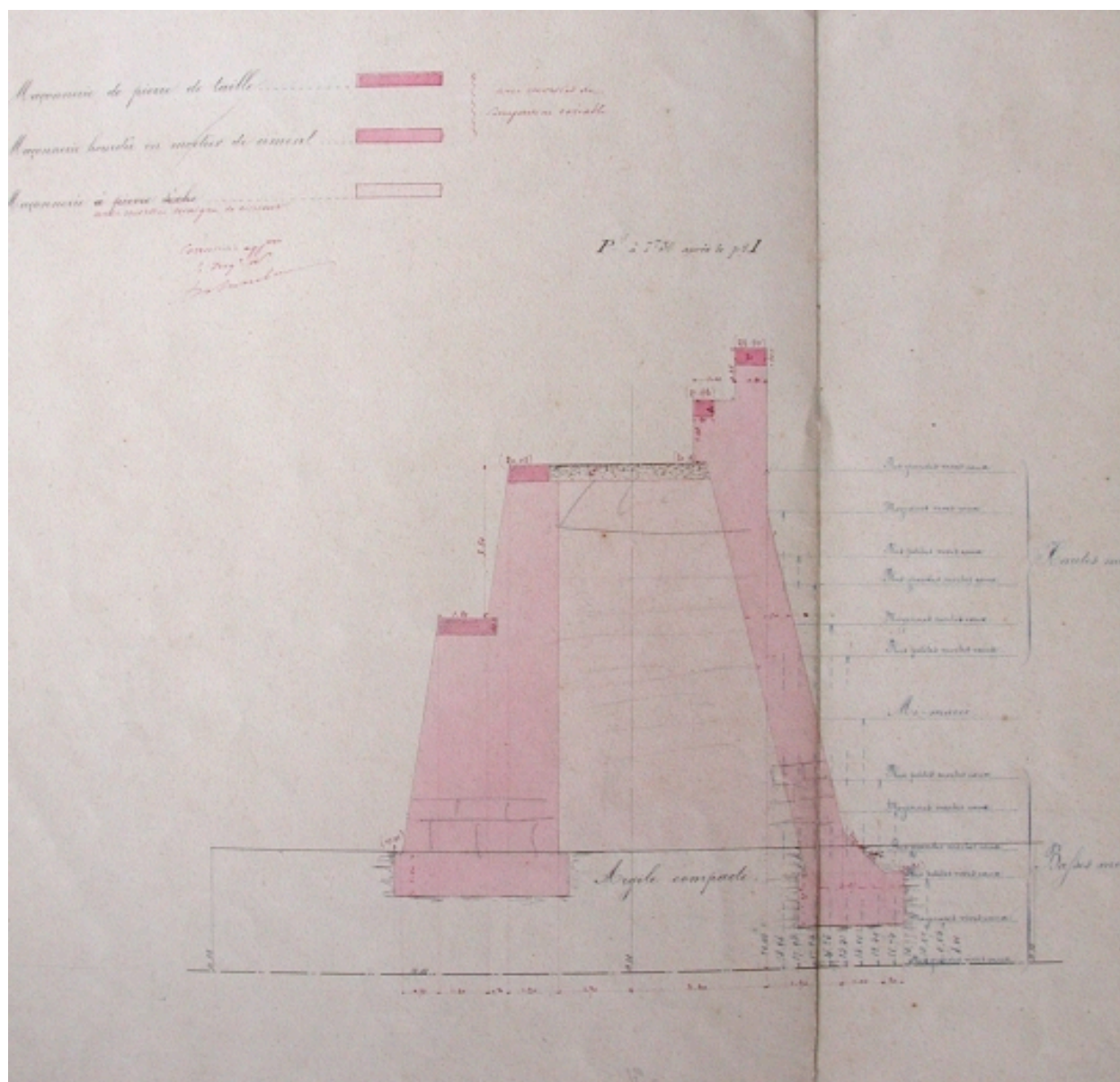
Projet de parapet sur la grande jetée en 1848 (AD 22)
