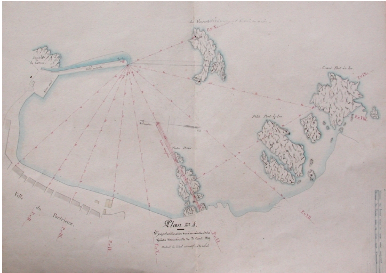
projet d'amélioration du port dressé en exécution en 1849 : Plan daté de 1849 : réalisation de la jetée du Tertre Denis, longue de 200 m (AD 22)
