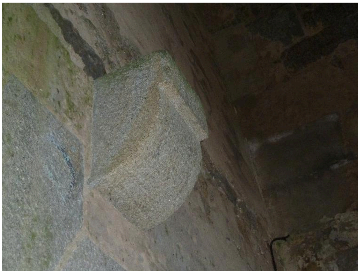
Hoedic, fort central, magasin à poudre, chambre de stockage, détail d'un corbeau du plancher de l'étage.
