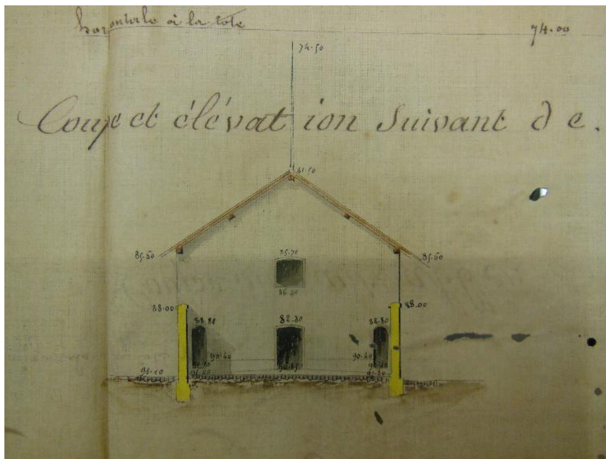
4 S3 5. Place de Houat-Hoedic, feuille n° 5 des projets pour 1855-1856, achever le fort d'Hoedic, magasin à poudre, 20 novembre 1854.
