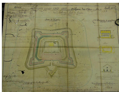
4 S3 5. Place de Houat-Hoedic, feuille n° 5 des projets pour 1855-1856, achever le fort d'Hoedic, magasin à poudre, 20 novembre 1854.
