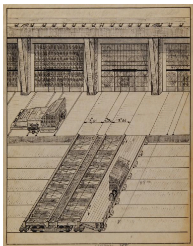
Dessin du chariot de translation avec ses quatre rails spéciaux et du tracteur-pousseur, croquis XII (Service Historique de la Défense de Lorient, Monographie de la base "Ingénieur Général Stoskopf", 1945-1946) Phot. Service Historique de la Défense IVR53_20225606364NUCA
